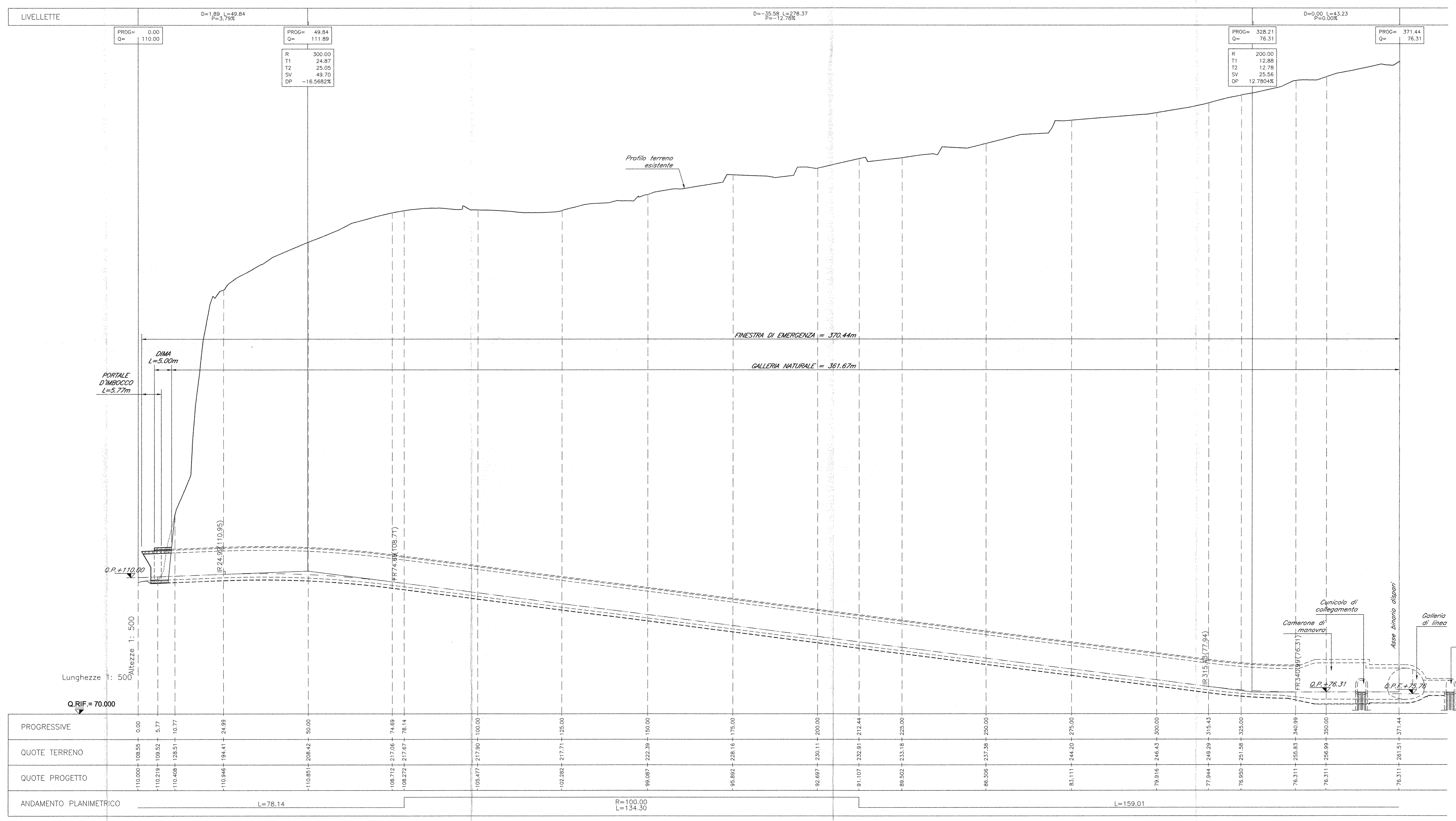
PROFLO LONGITUDINALE IN ASSE FINESTRA DI EMERGENZA scala 1:500
