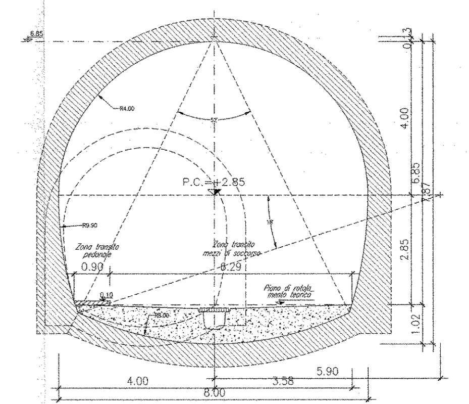
SEZIONE D-D SCALA 1:100 ALLARGO PER INCROCIO MEZZI
