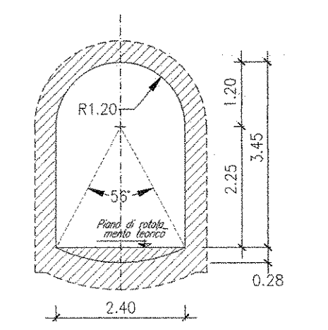
SEZIONE C-C SCALA 1:100 CUNICOLO DI COLLEGAMENTO ALLA FINESTRA
