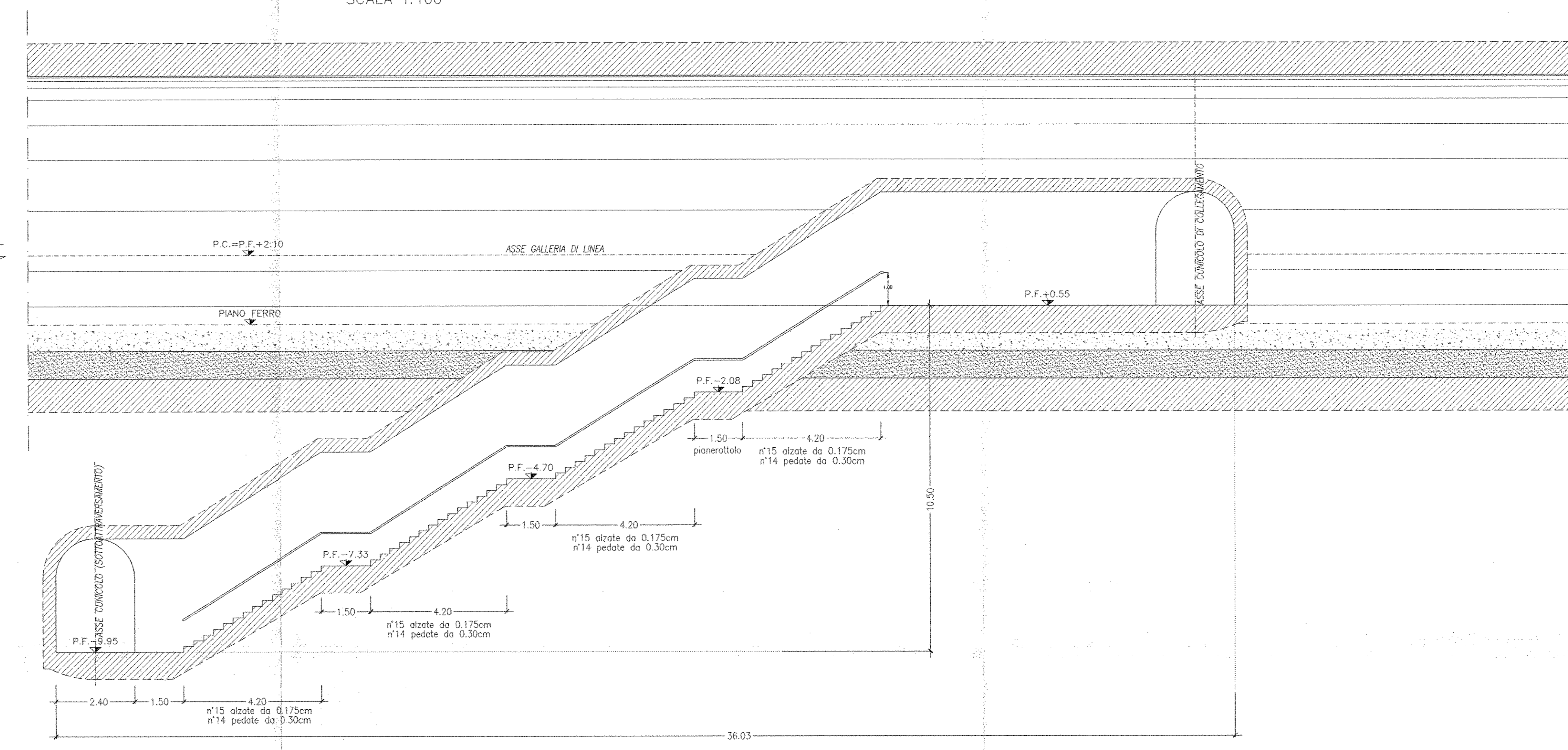
SEZIONE 3-3 SCALA 1:100
