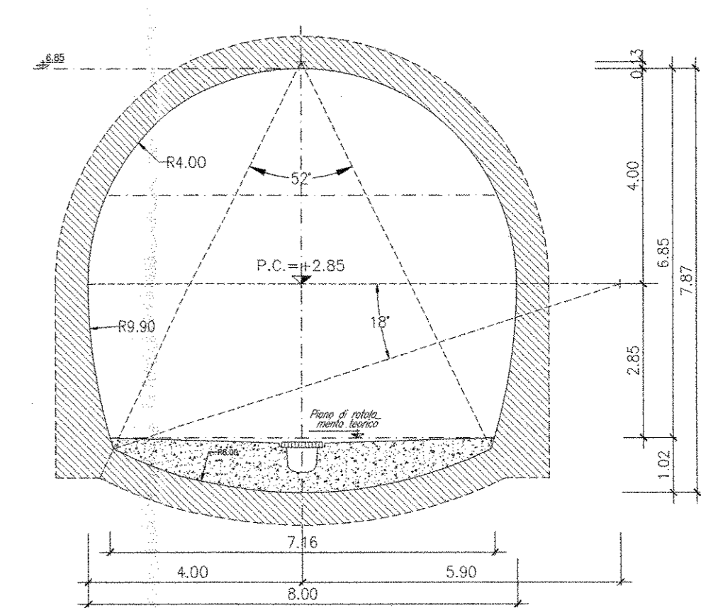
SEZIONE A-A SCALA 1:100 CAMERA DI MANOVRA
