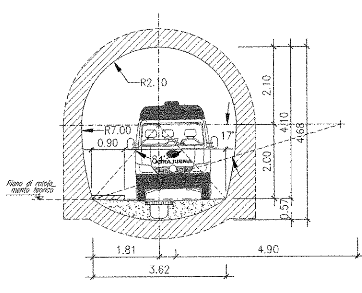
SEZIONE B-B SCALA 1:100 CUNICOLO DI SFOLLAMENTO
