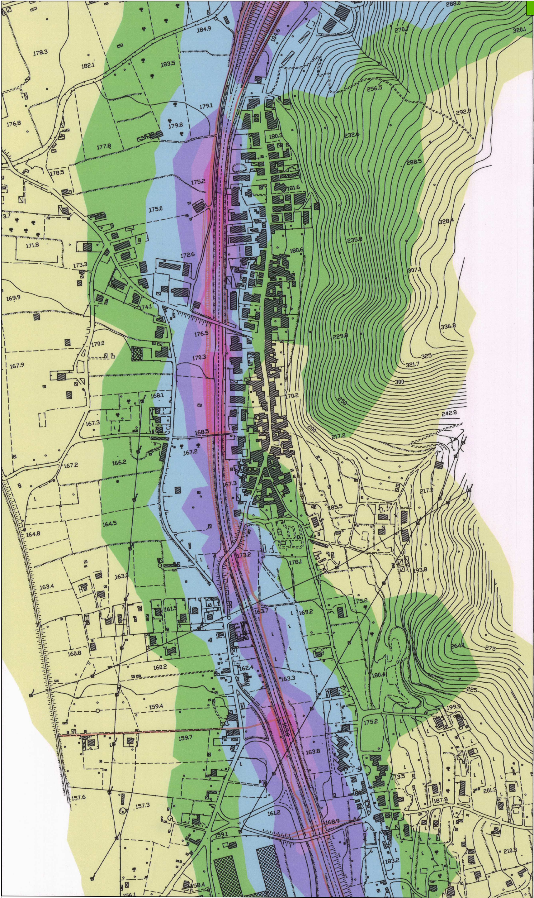
Livelli di pressione sonora Leq(A)
