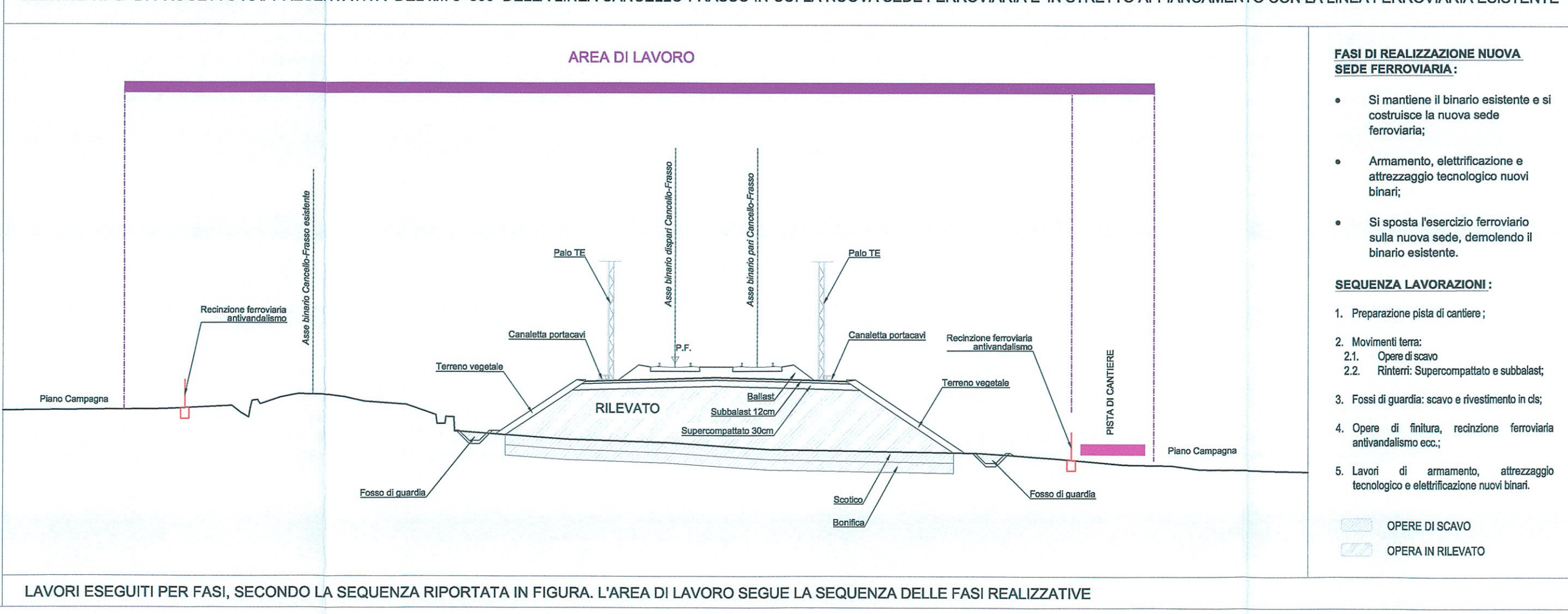
*SEZIONE TIPO* DI PROGETTO RAPPRESENTATIVA DEL km 8+500 DELLA LINEA CANCELLO-FRASSO IN CUI LA NUOVA SEDE FERROVIARIA E' IN STRETTO AFFIANCAMENTO CON LA LINEA FERROVIARIA ESISTENTE
