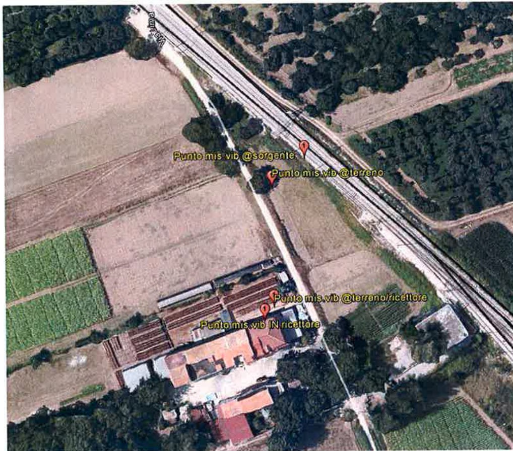
Localizzazione delle terne accelerometriche in corrispondenza della sezione dei rilievi vibrazionali
