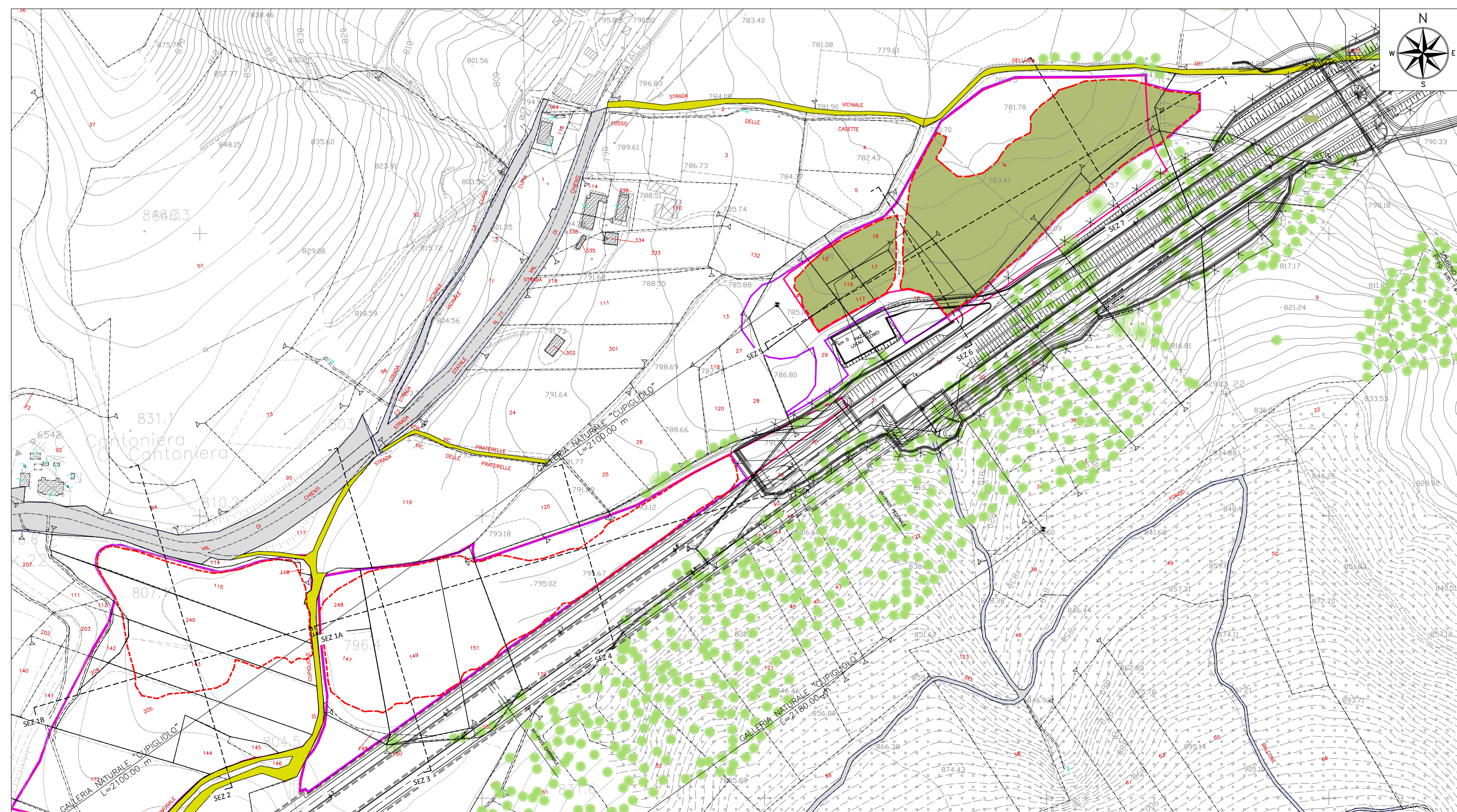
PLANIMETRIA DI PROGETTO - SCALA 1:2000
