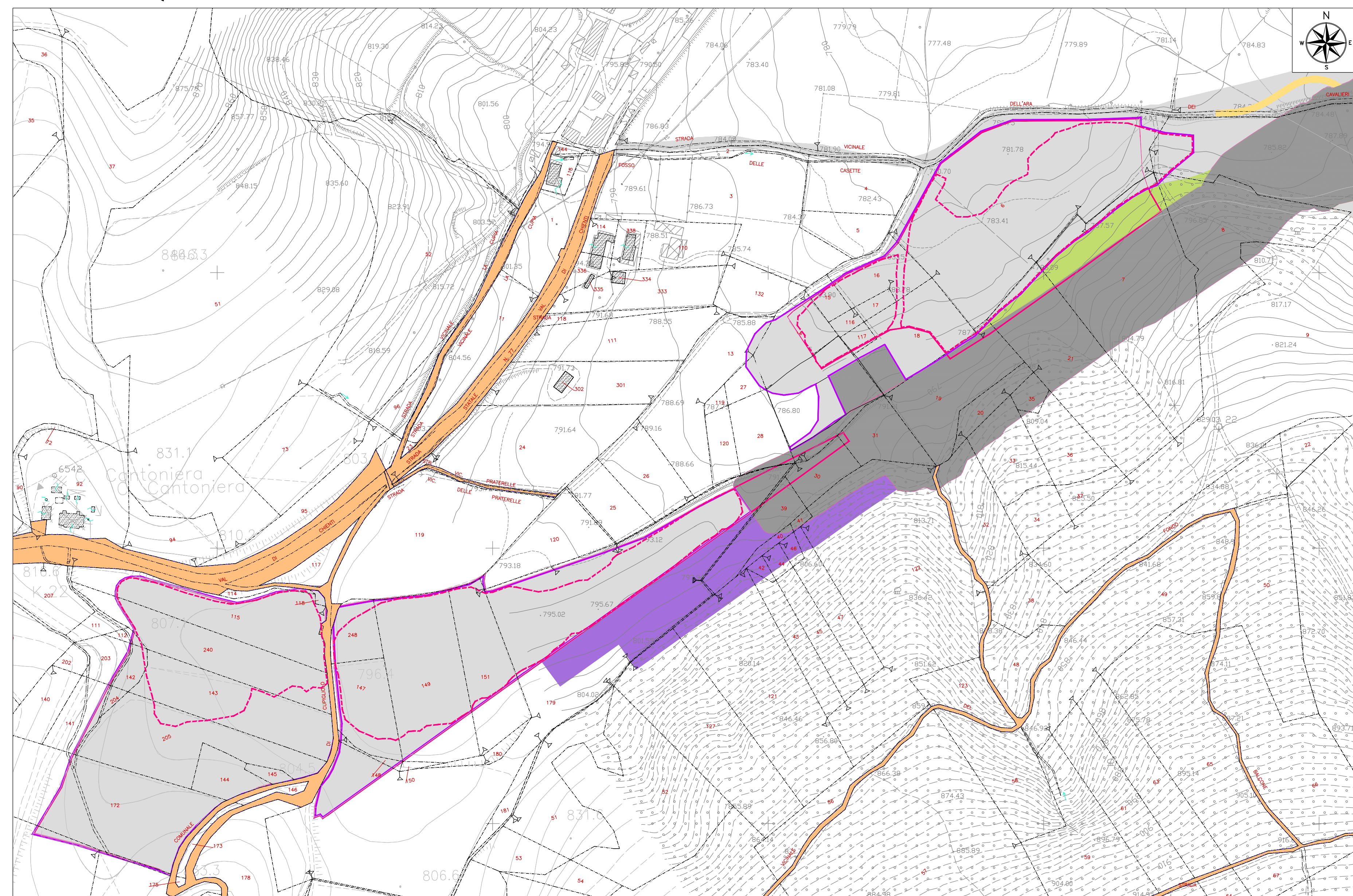
STRALCIO CATASTALE - SCALA 1:2000
