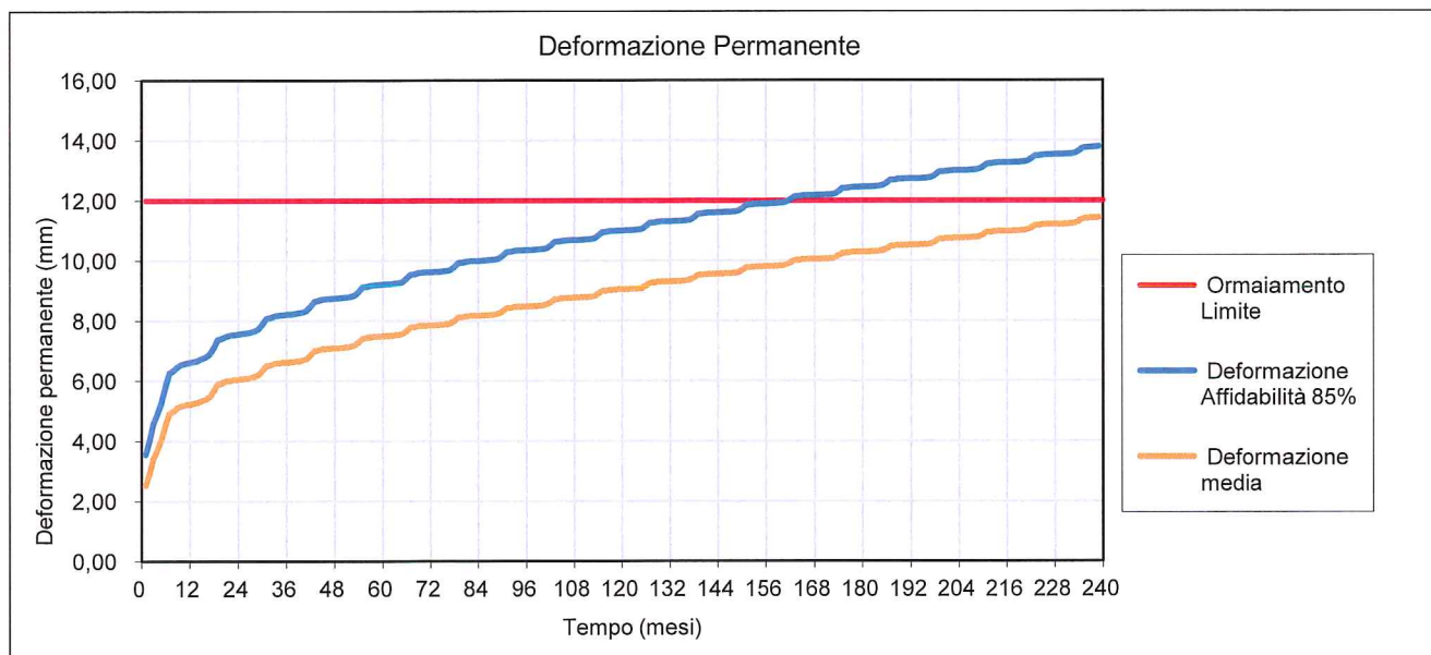
Figura 2 - Andamento della deformazione permanente nel pacchetto tipo B
