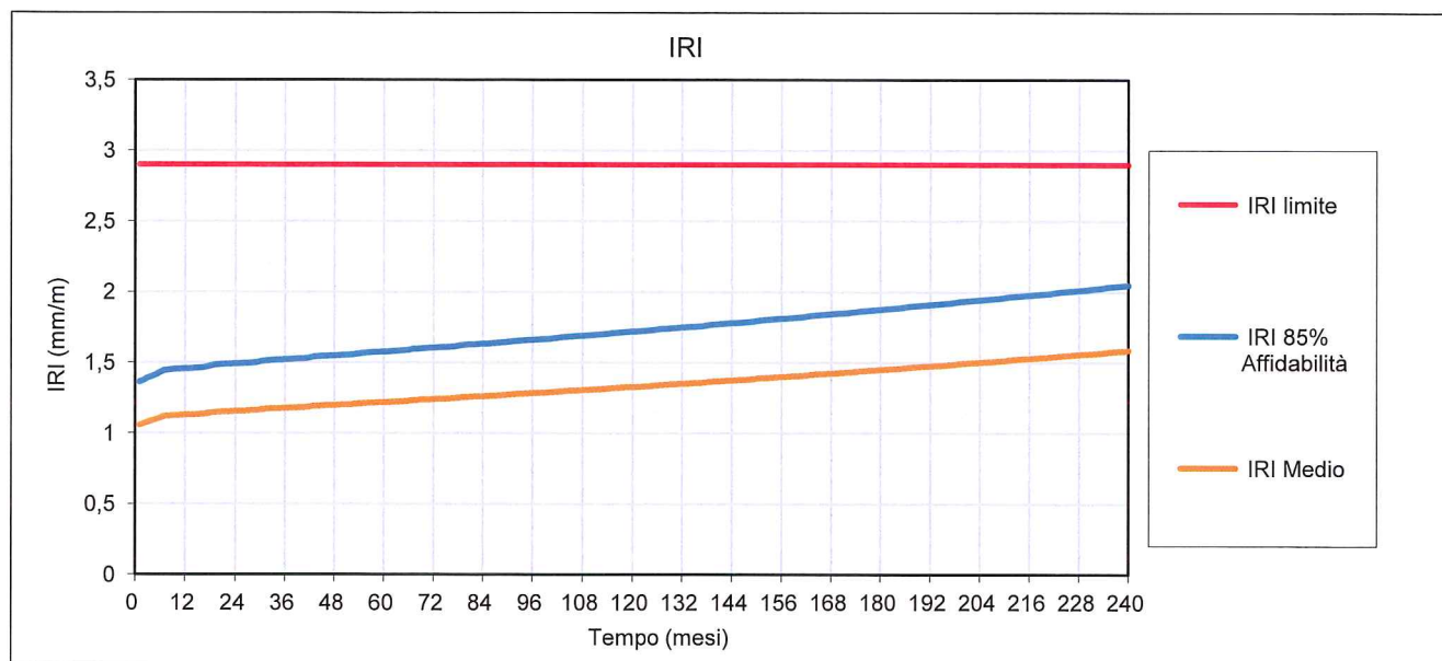
Figura 3 - Andamento della irregolarità longitudinale (indice IRI) nel pacchetto tipo B
