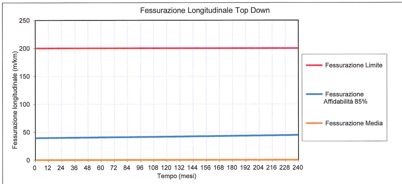
Figura 1 - Andamento della fessurazione longitudinale "top-down" nella pacchetto tipo B
