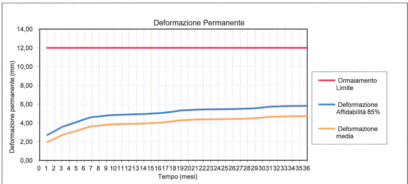
Figura 2 - Andamento della deformazione permanente nel pacchetto tipo F
