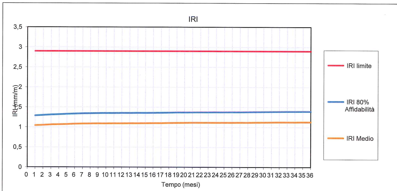
Figura 3 - Andamento della irregolarità longitudinale (indice IRI) nel pacchetto tipo F
