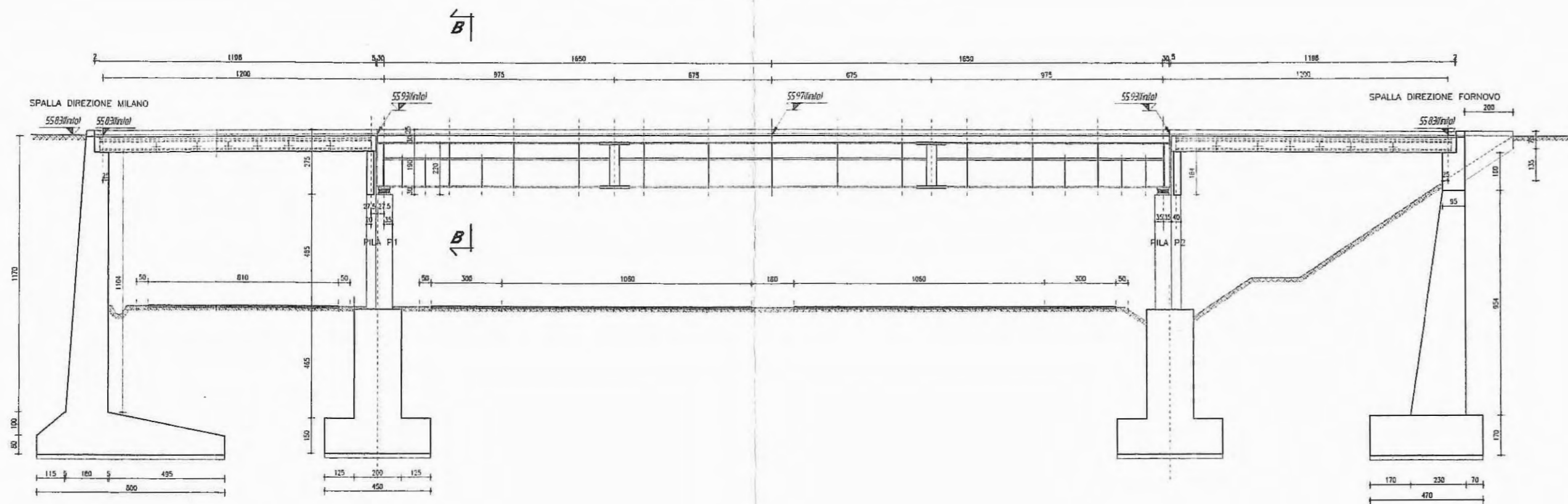
SEZIONE A-A
