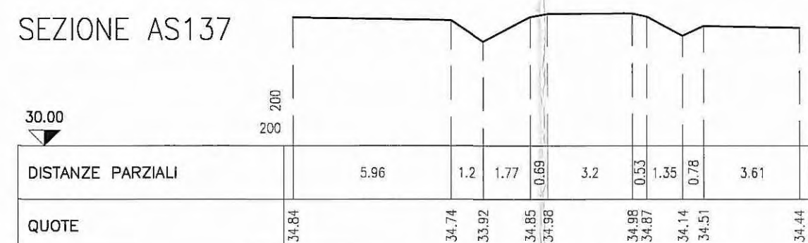
SEZIONE AS137
