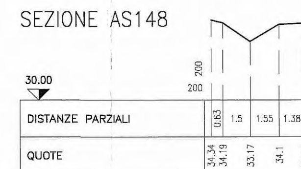
SEZIONE AS148
