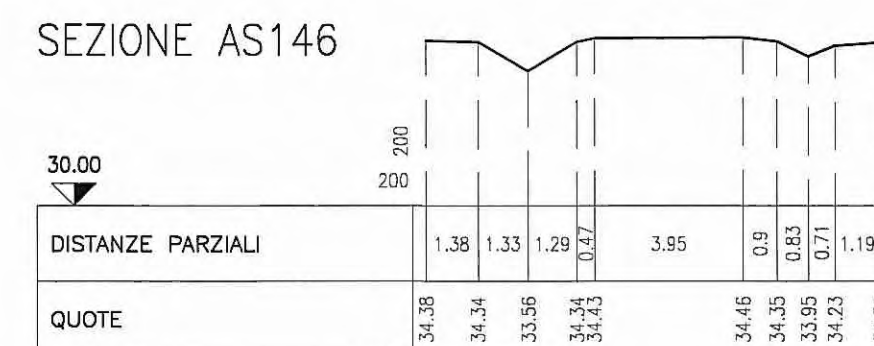
SEZIONE AS146
