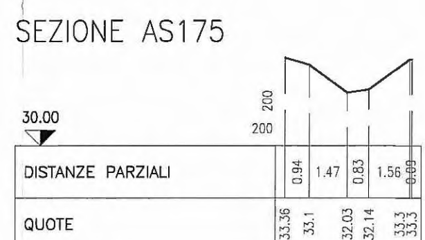
SEZIONE AS175
