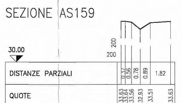
SEZIONE AS159
