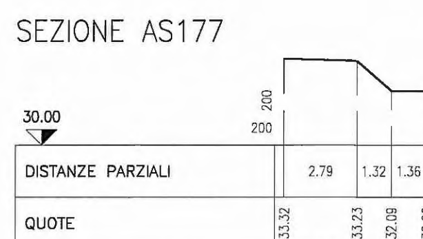
SEZIONE AS177
