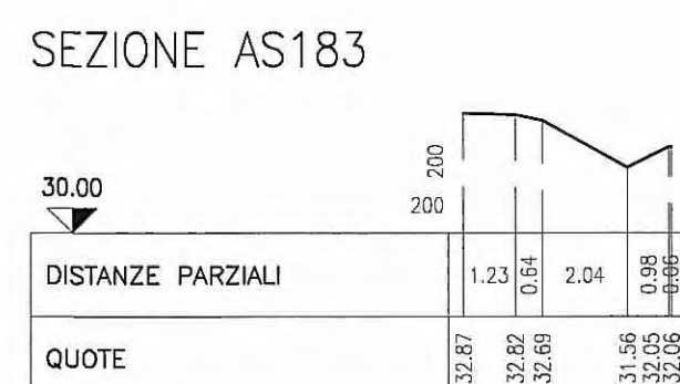
SEZIONE AS183
