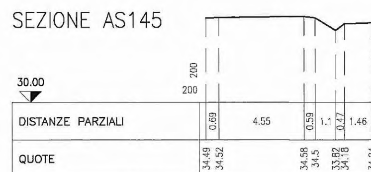
SEZIONE AS145
