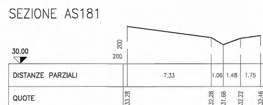
SEZIONE AS181
