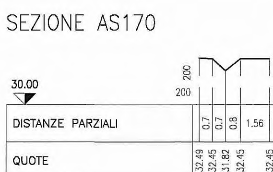
SEZIONE AS170
