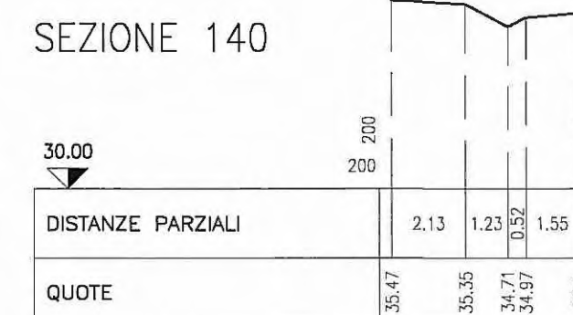
SEZIONE 140
