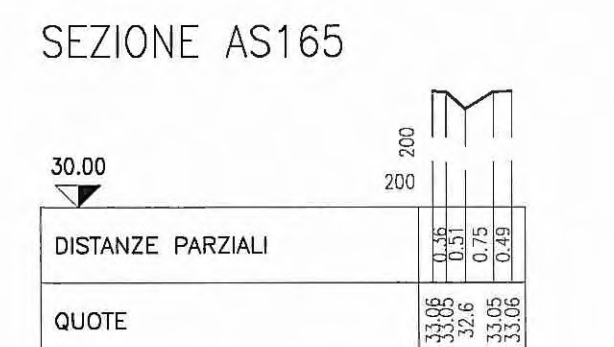
SEZIONE AS165
