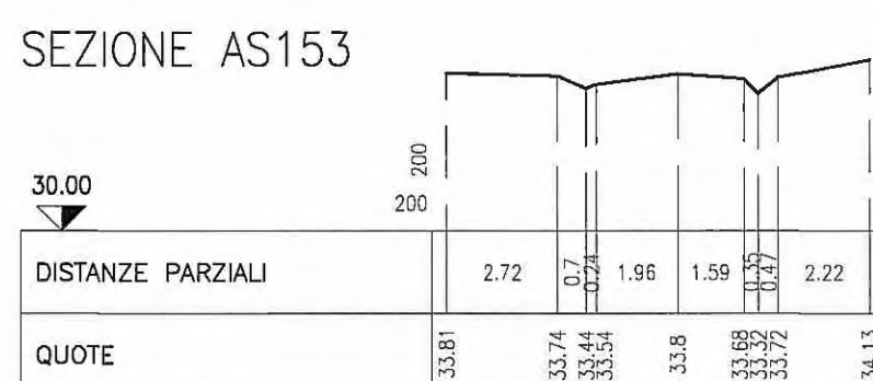
SEZIONE AS153
