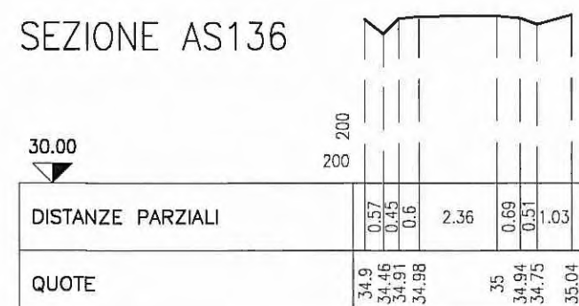
SEZIONE AS136
