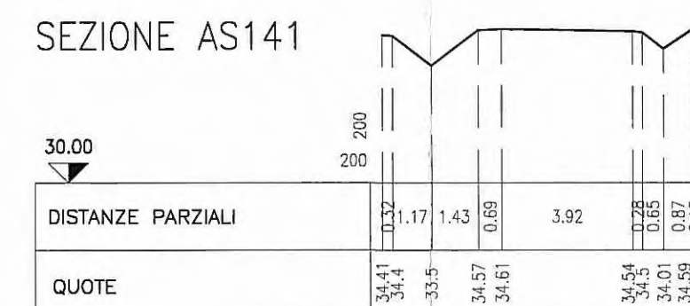
SEZIONE AS141
