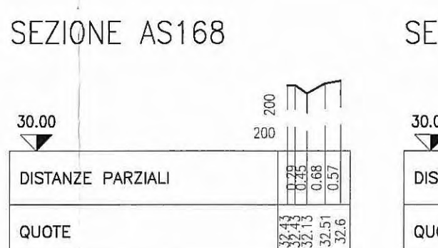
SEZIONE AS168
