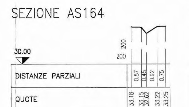
SEZIONE AS164
