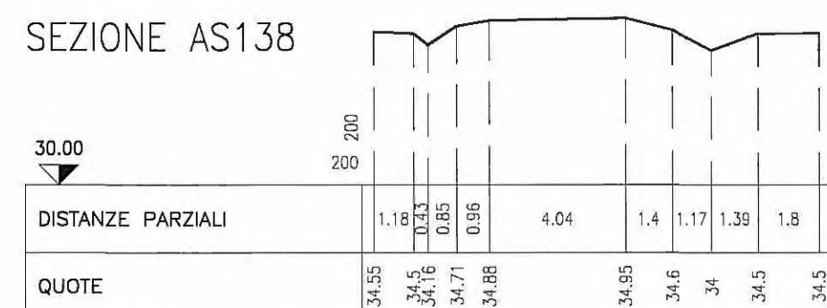
SEZIONE AS138
