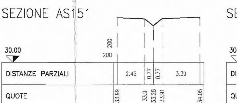
SEZIONE AS151
