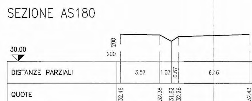
SEZIONE AS180
