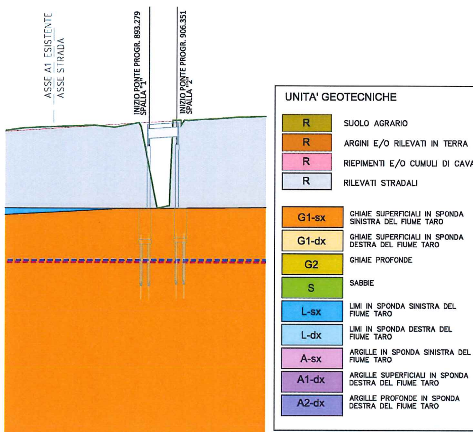
Fig. 6.2 Profilo Geotecnico
