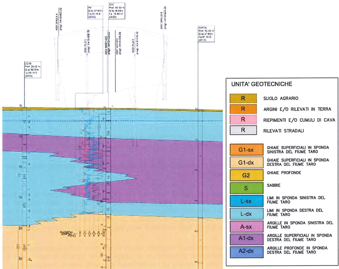
Fig. 6.2 Profilo Geotecnico
