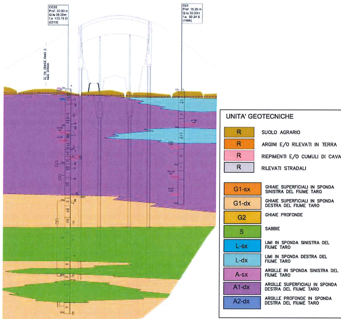
Fig. 6.2 Profilo Geotecnico
