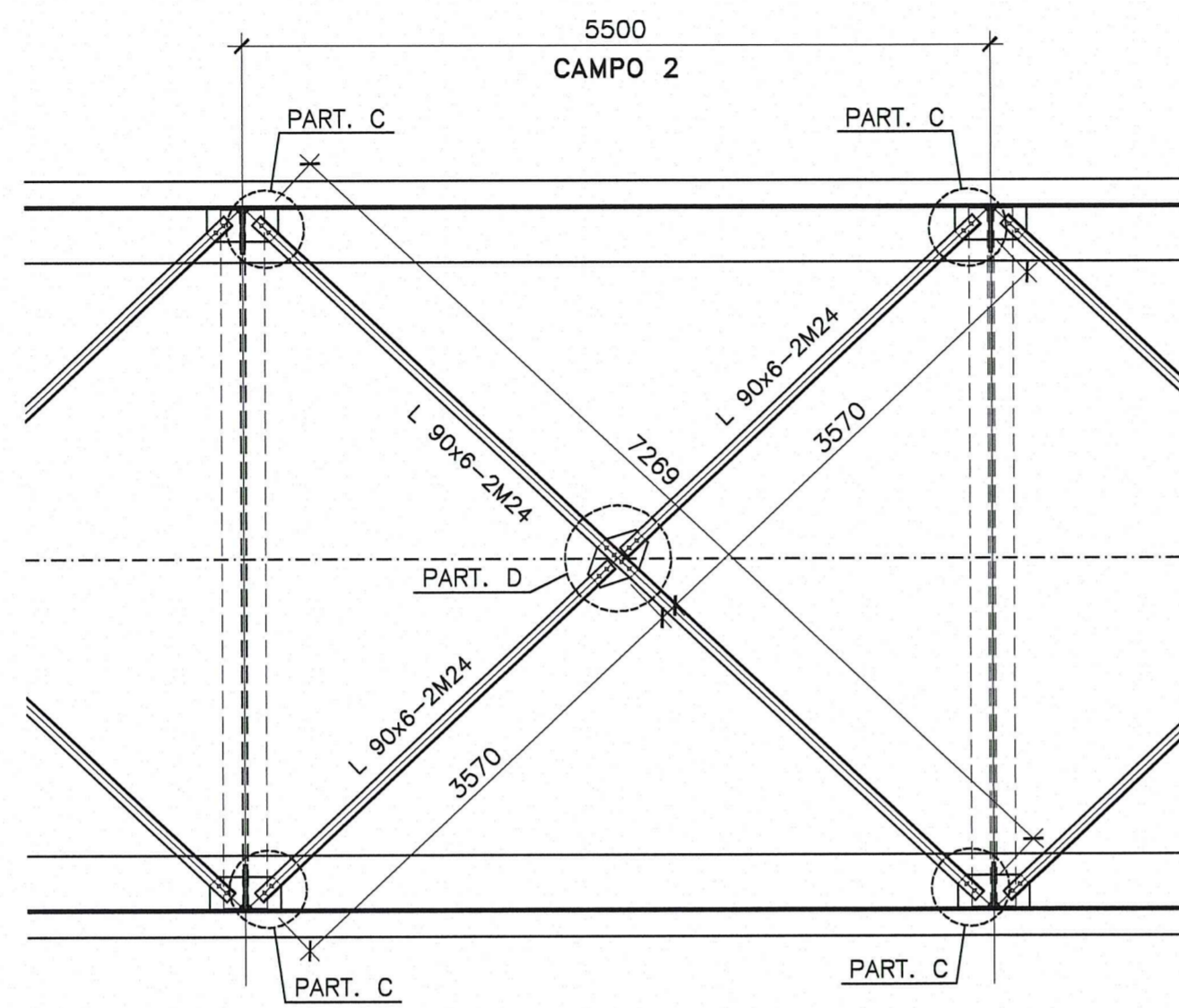
CONTROVENTI CAMPO 2 SCALA 1:50
