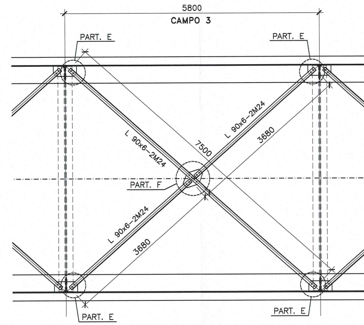
CONTROVENTI CAMPO 3 SCALA 1:50
