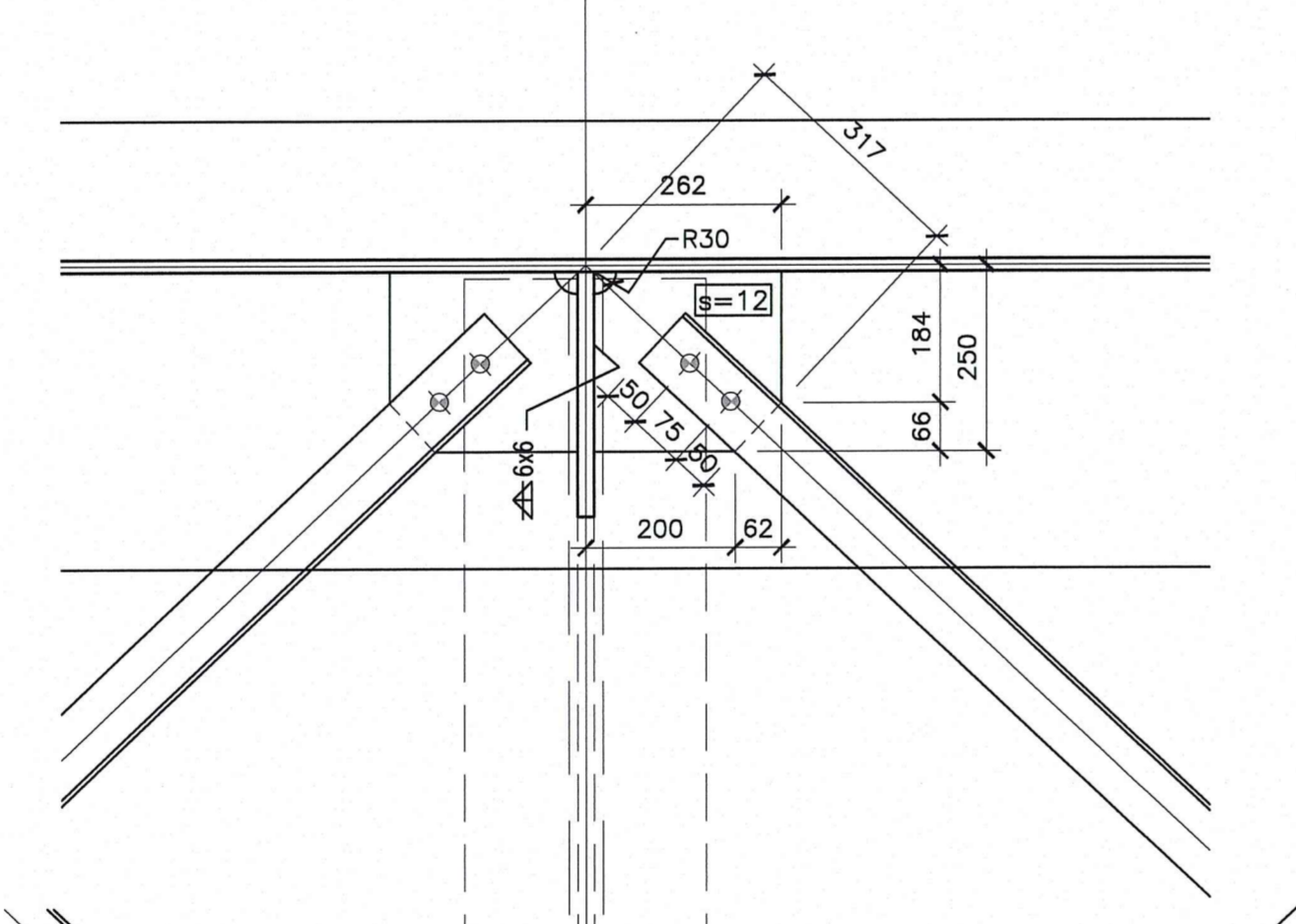
PARTICOLARE C SCALA 1:10
