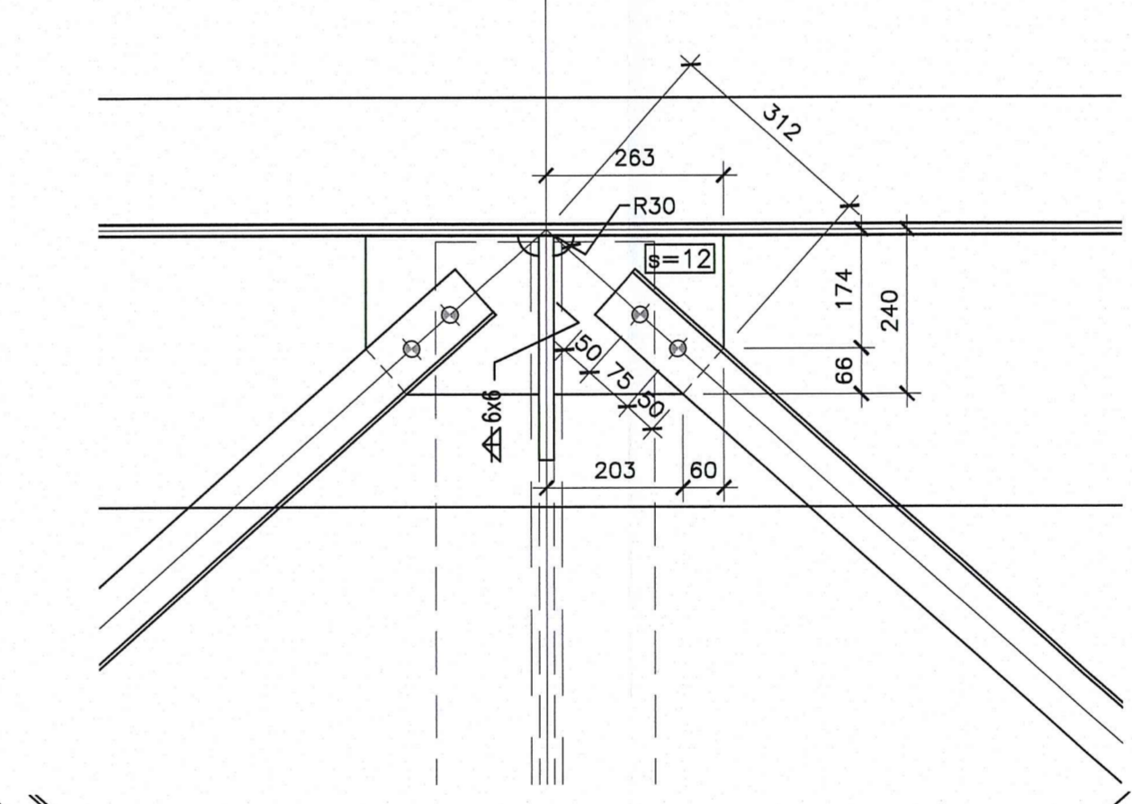
PARTICOLARE E SCALA 1:10
