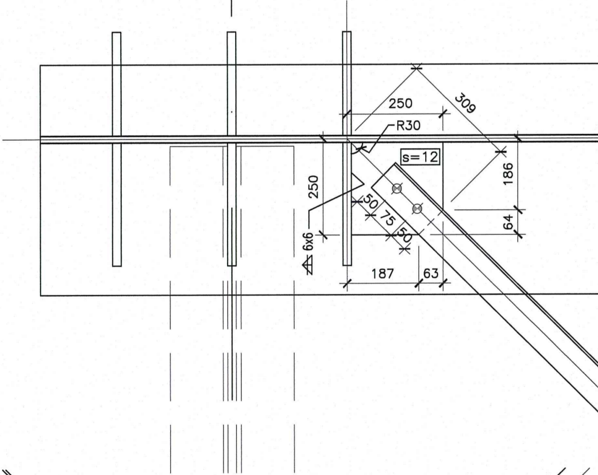
PARTICOLARE A SCALA 1:10
