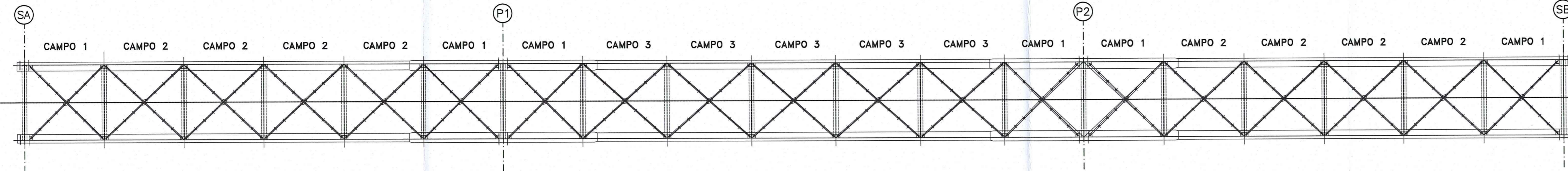
CONTROVENTI CAMPO 1 SCALA 1:50
