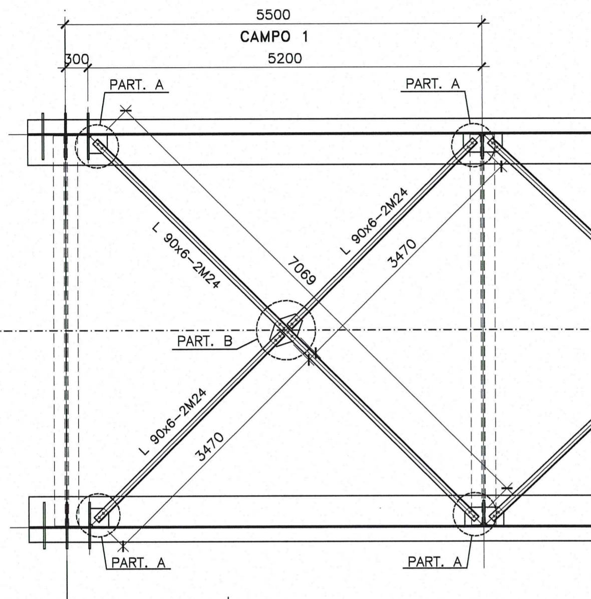
CONTROVENTI CAMPO 1 SCALA 1:50
