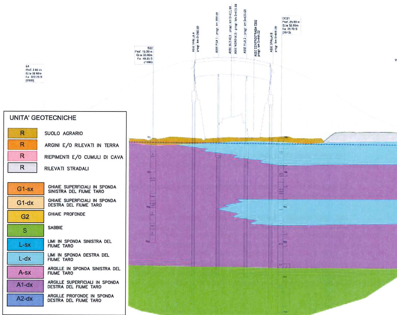
Fig. 6.2 Profilo Geotecnico
