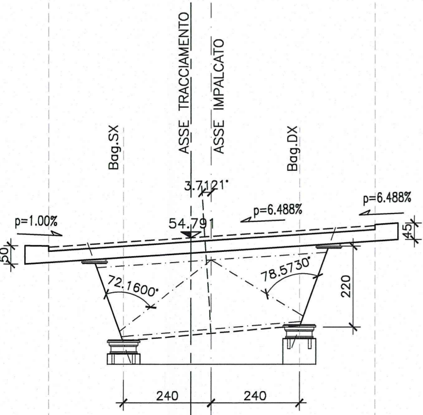
PILA 3
