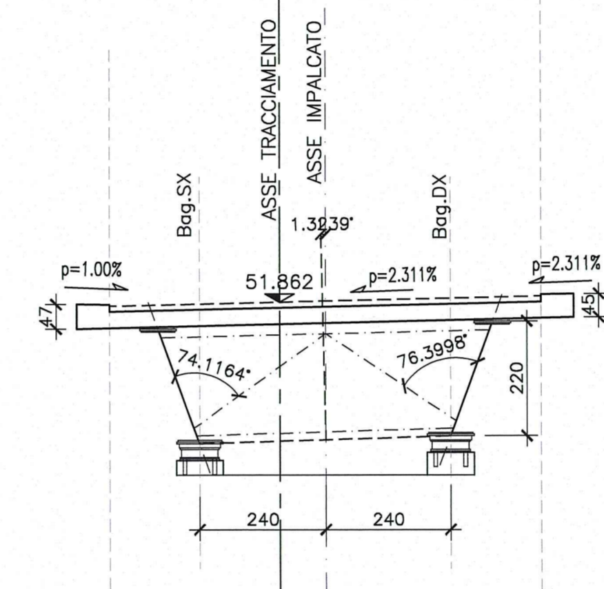
PILA 9
