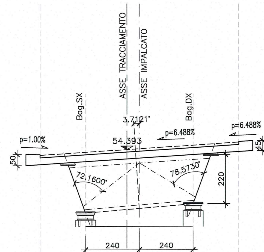
PILA 7
