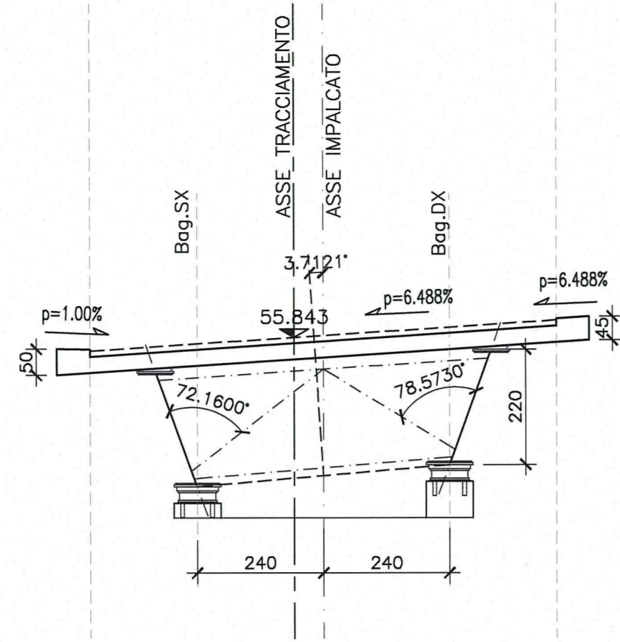
PILA 4
