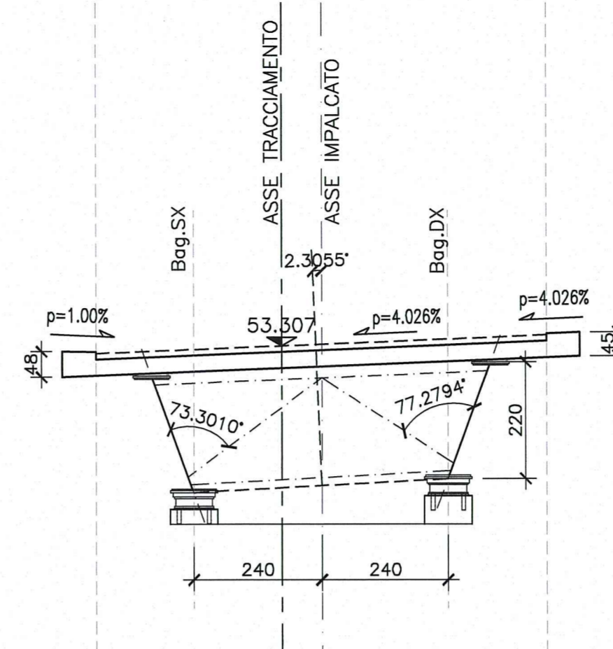
PILA 8
