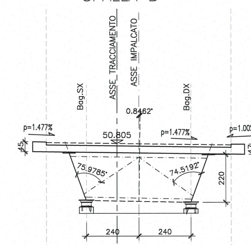
SPALLA B
