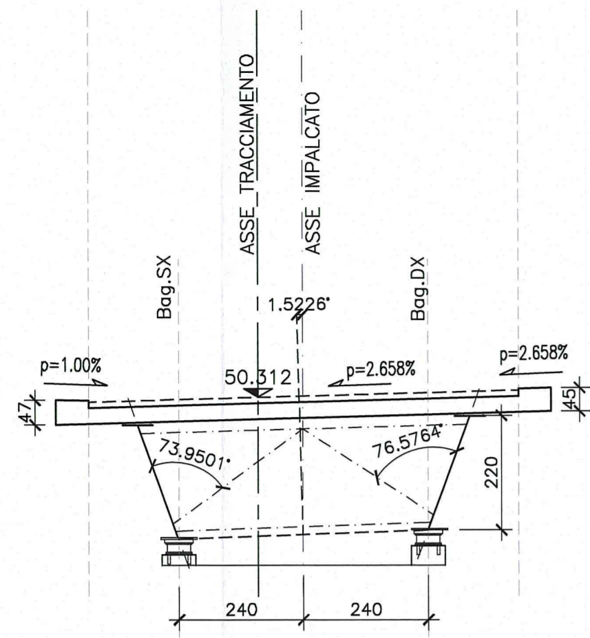
SPALLA A
