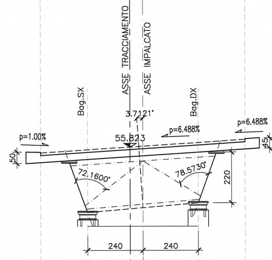
PILA 5
