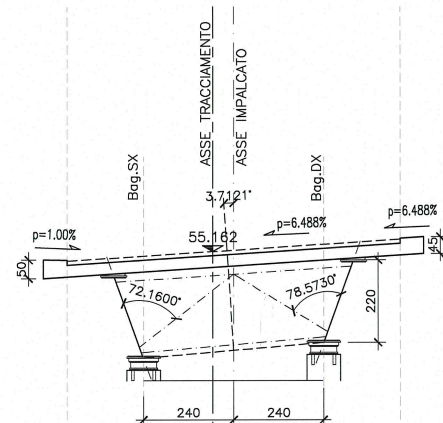
PILA 6
