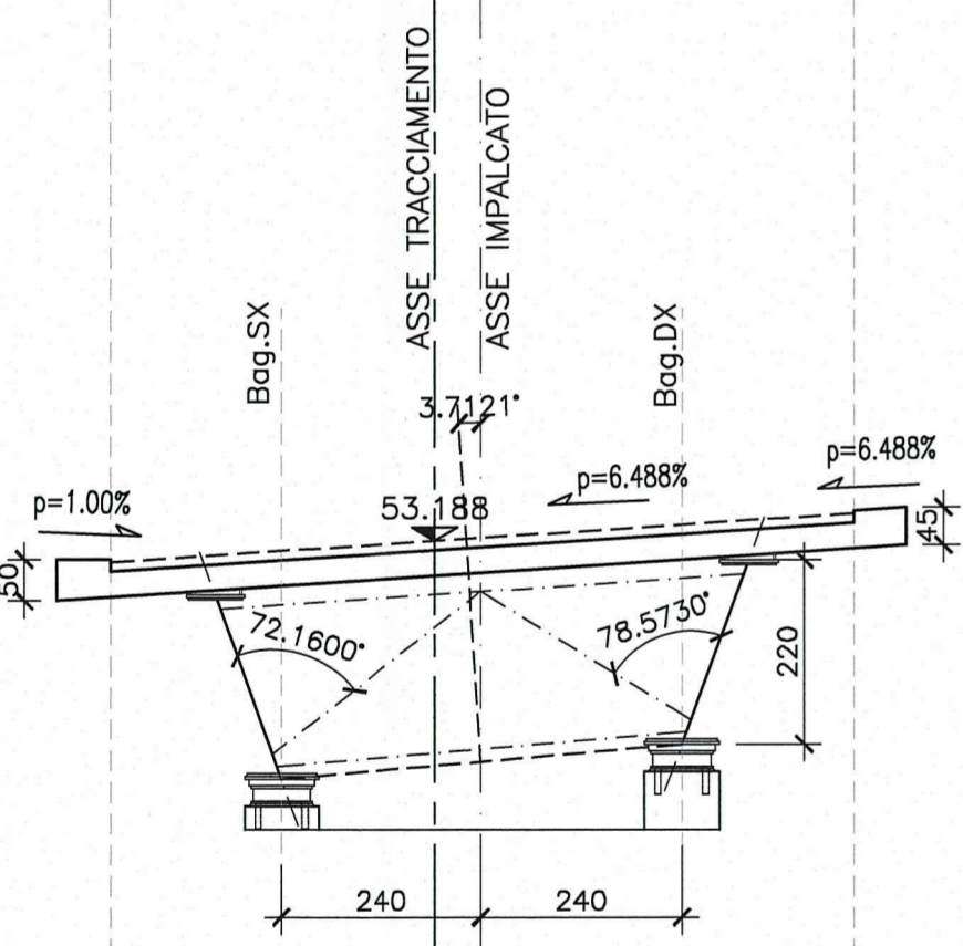
PILA 2
