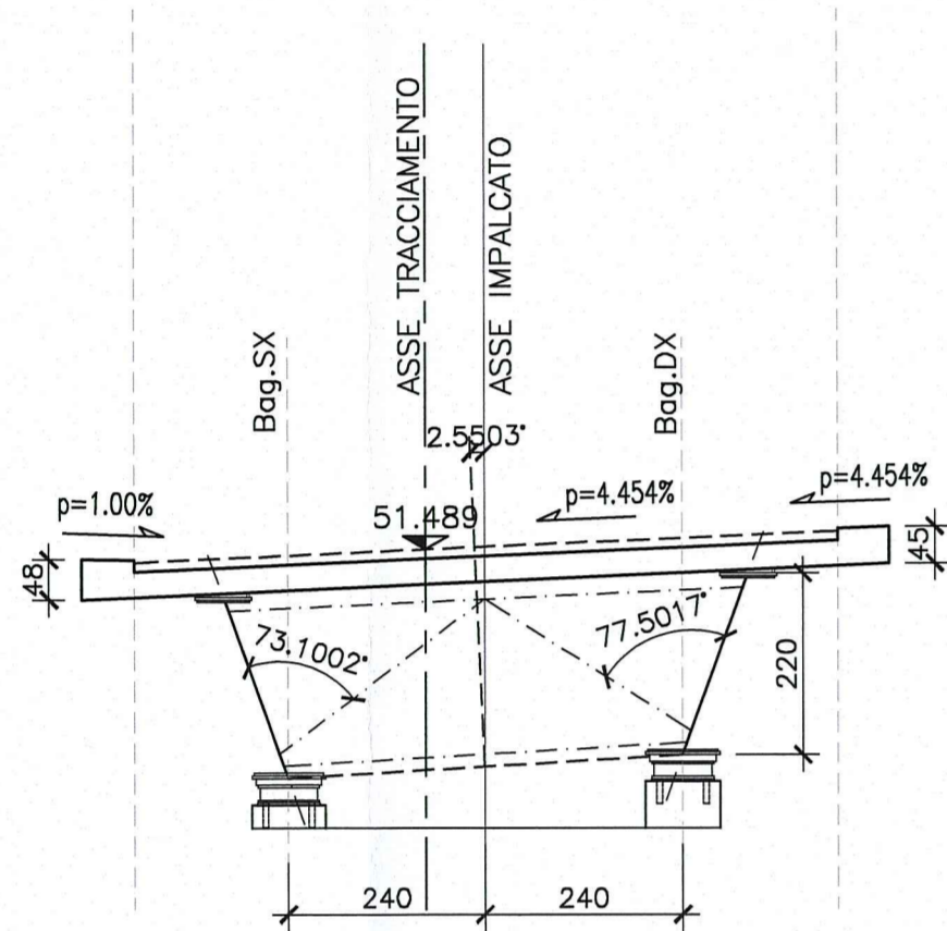
PILA 1
