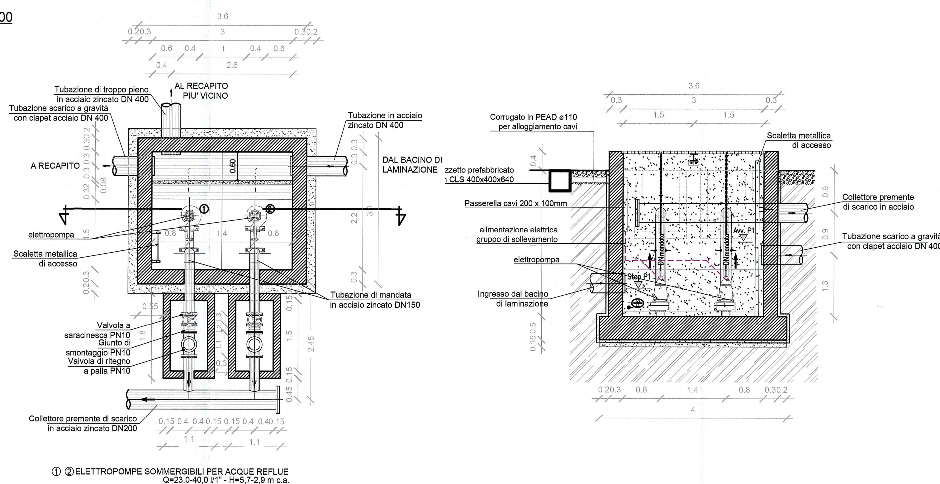
① ② ELETTROPOMPE SOMMERSIBILI PER ACQUE REFLUE Q=23,0-40,0 l/s - H=5,7-2,9 m c.a.
