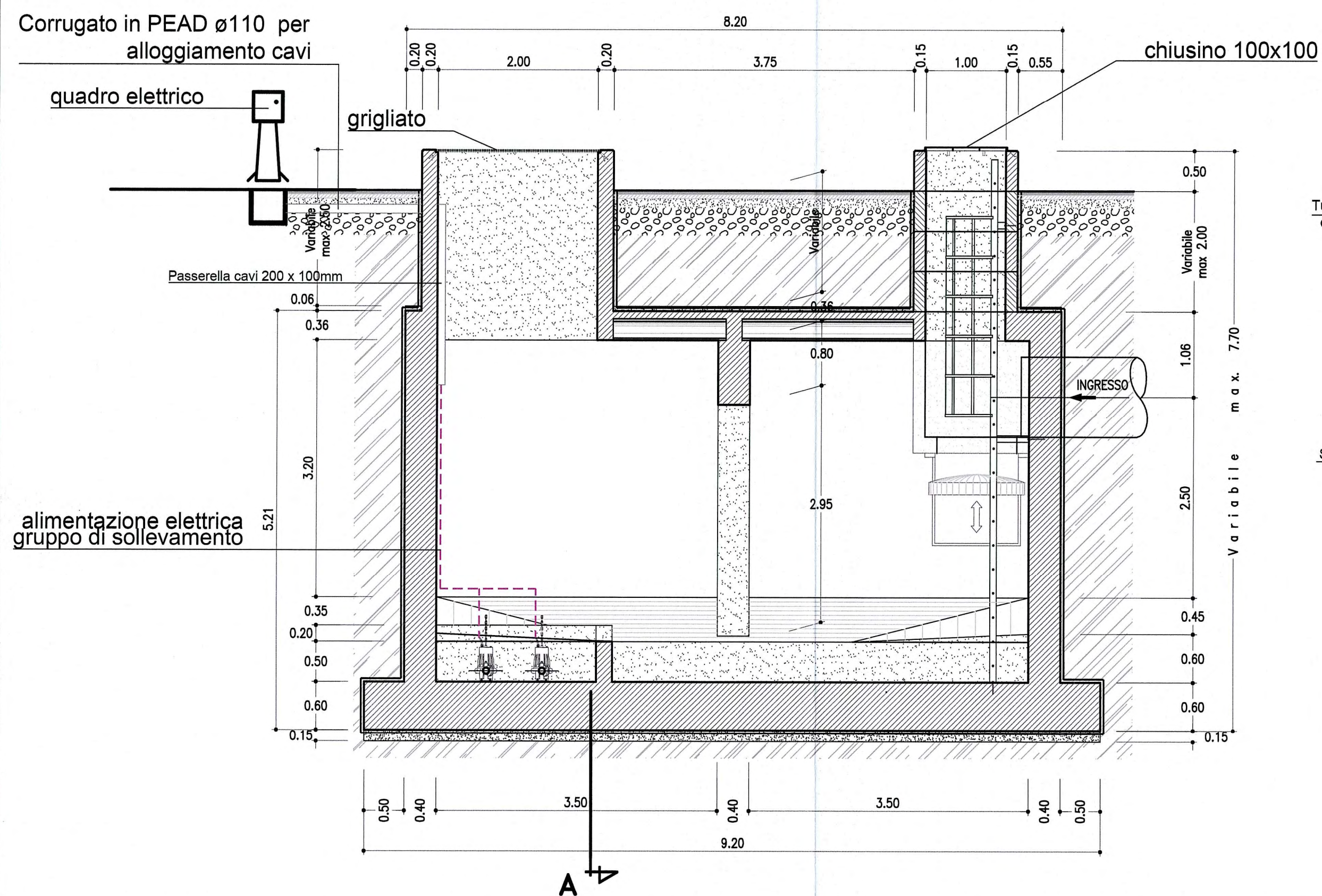
Vasca di prima pioggia - vista in sezione scala 1:50
