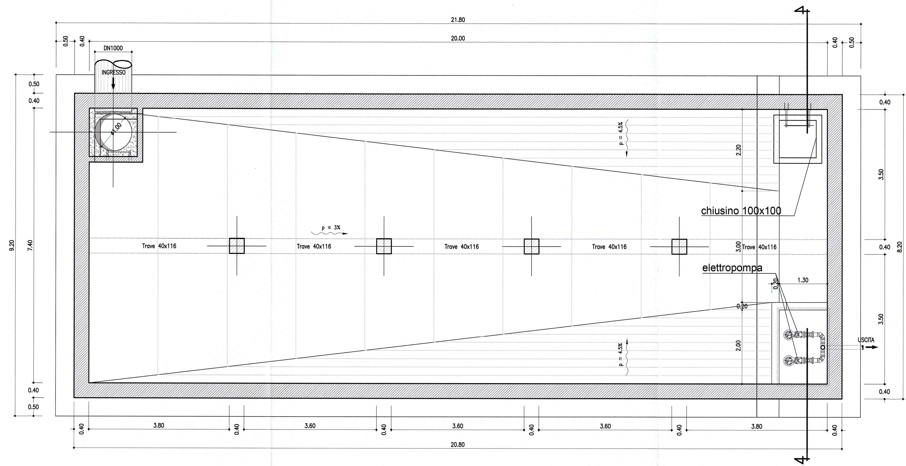
Vasca di prima pioggia - vista in pianta scala 1:50
