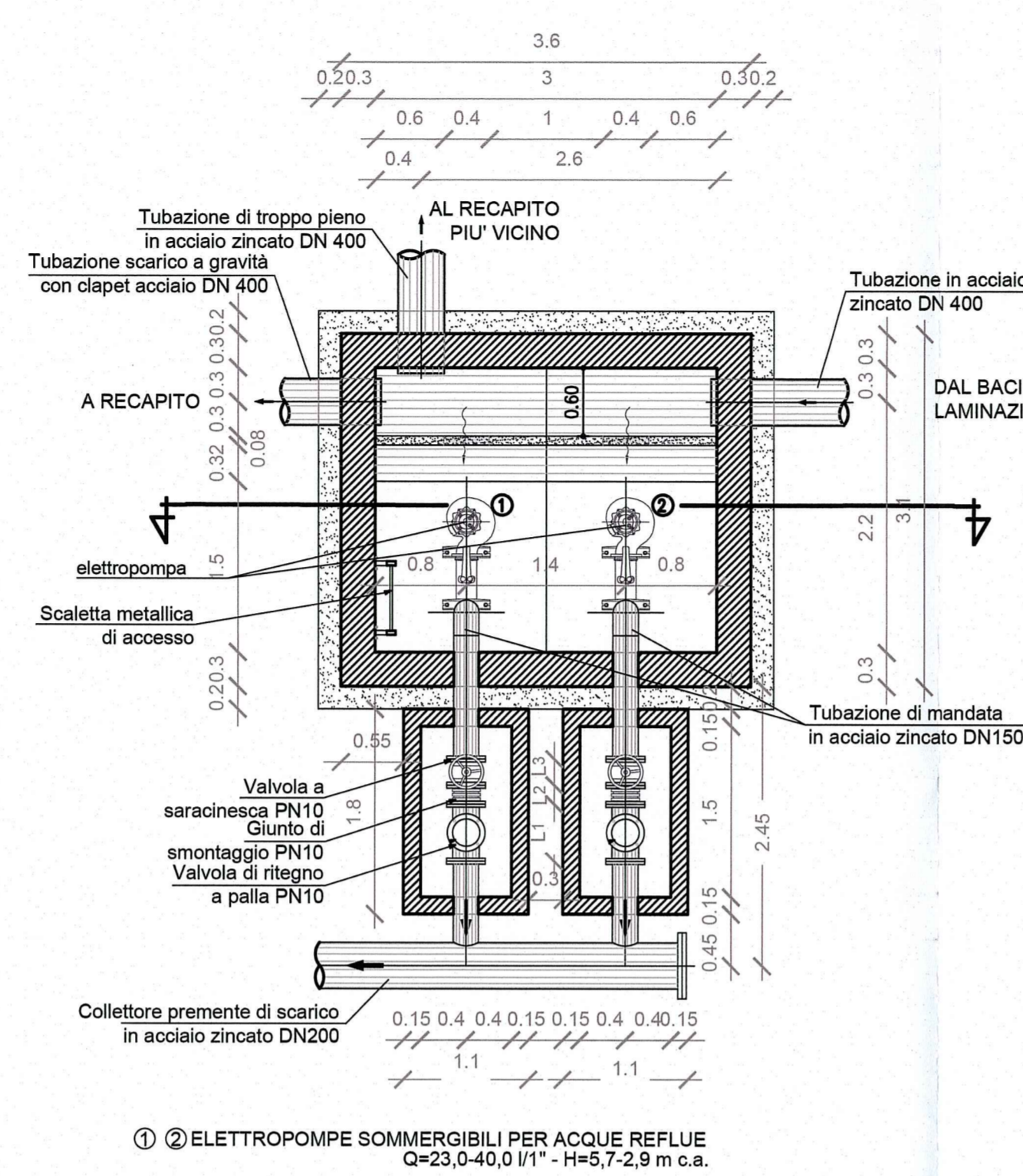
Impianto di sollevamento - vista in pianta scala 1:50
