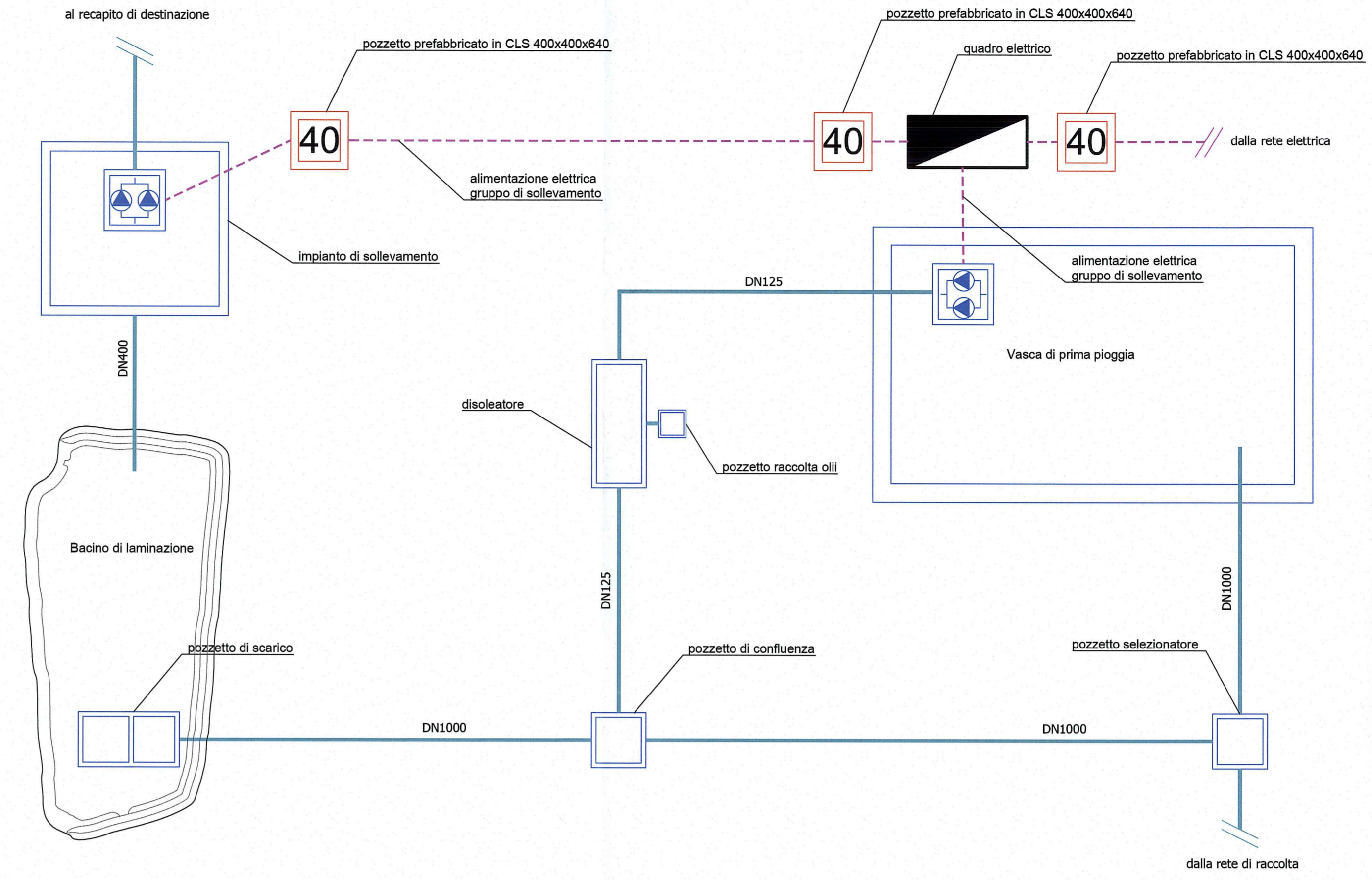
Schema di funzionamento dell'impianto trattamento acque
