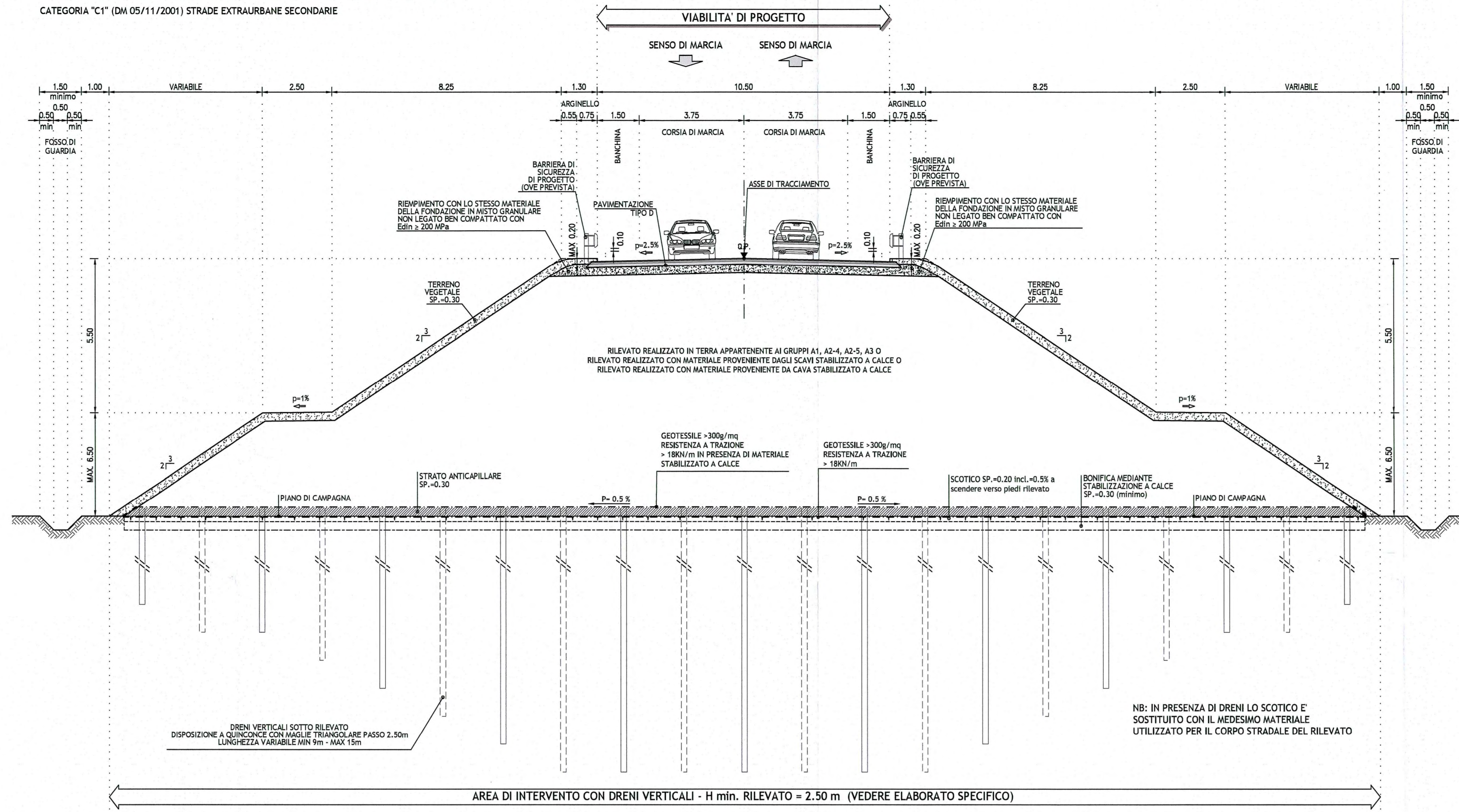
Tipo 1b in curva VIABILITA' INTERFERENTE IN CURVA CON RILEVATO H < 5.50m - scala 1:100 CATEGORIA "C1" (DM 05/11/2001) STRADE EXTRAURBANE SECONDARIE
