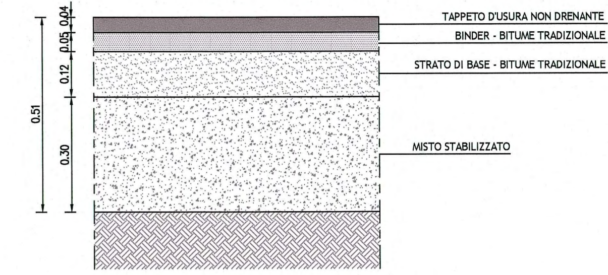
Pacchetto stradale PAVIMENTAZIONE TIPO "D" scala 1:10
