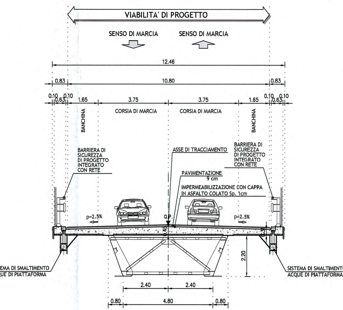
Tipo 2a su cavalcavia IN RETTILINEO - scala 1:100 CATEGORIA "C1" (DM 05/11/2001) STRADE EXTRAURBANE SECONDARIE SEZIONE TIPO IN CAMPATA CAVALCAVIA "CA.08"
