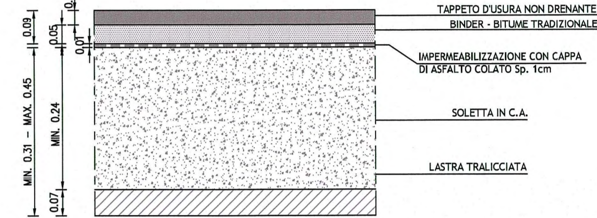
Pacchetto su opera d'arte scala 1:10 PAVIMENTAZIONE CAVALCAVIA "CA.08"
