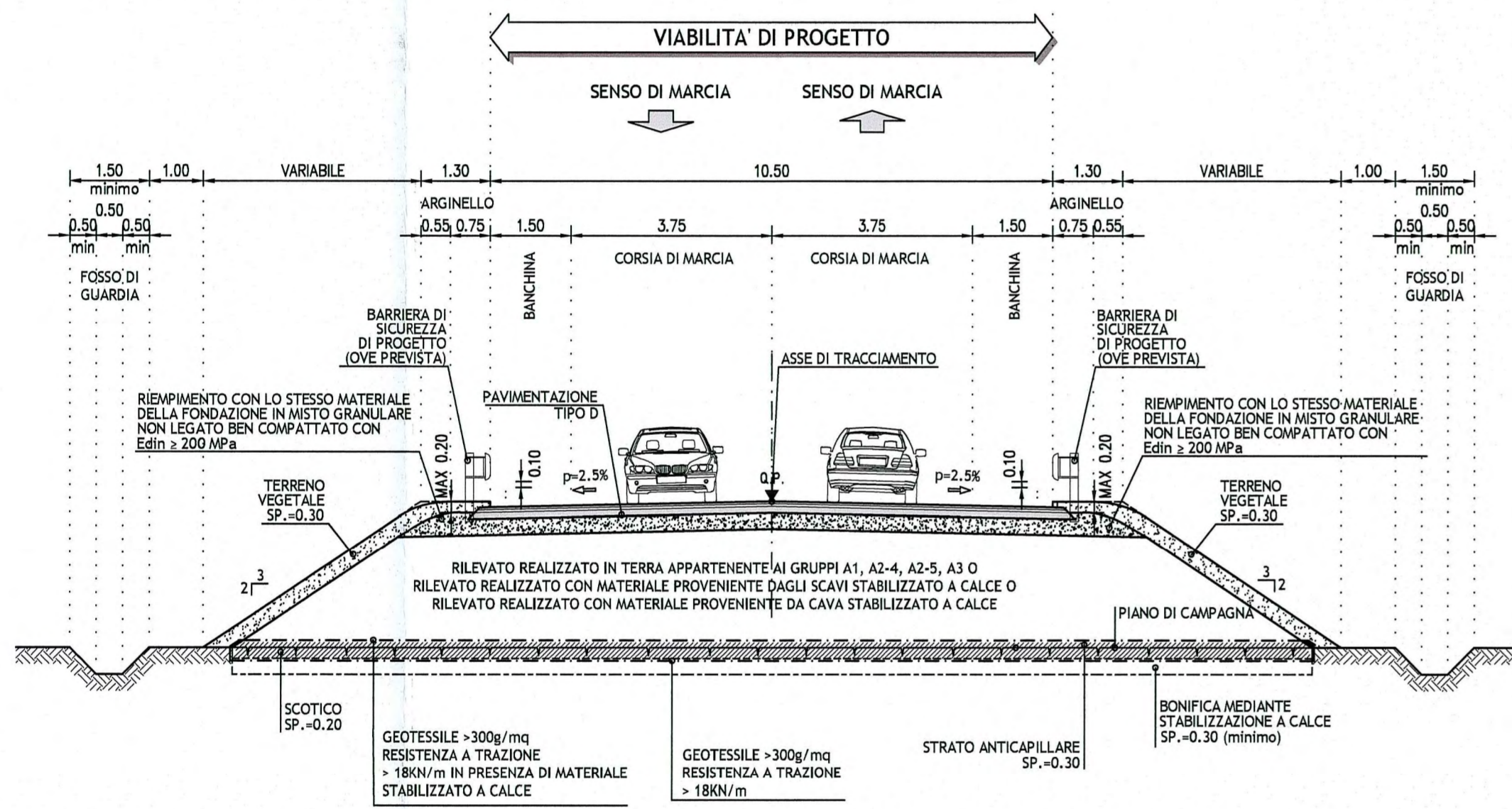
Tipo 1a in rilevato VIABILITA' INTERFERENTE IN RETTILINEO CON RILEVATO H < 5.50m - scala 1:100 CATEGORIA "C1" (DM 05/11/2001) STRADE EXTRAURBANE SECONDARIE
