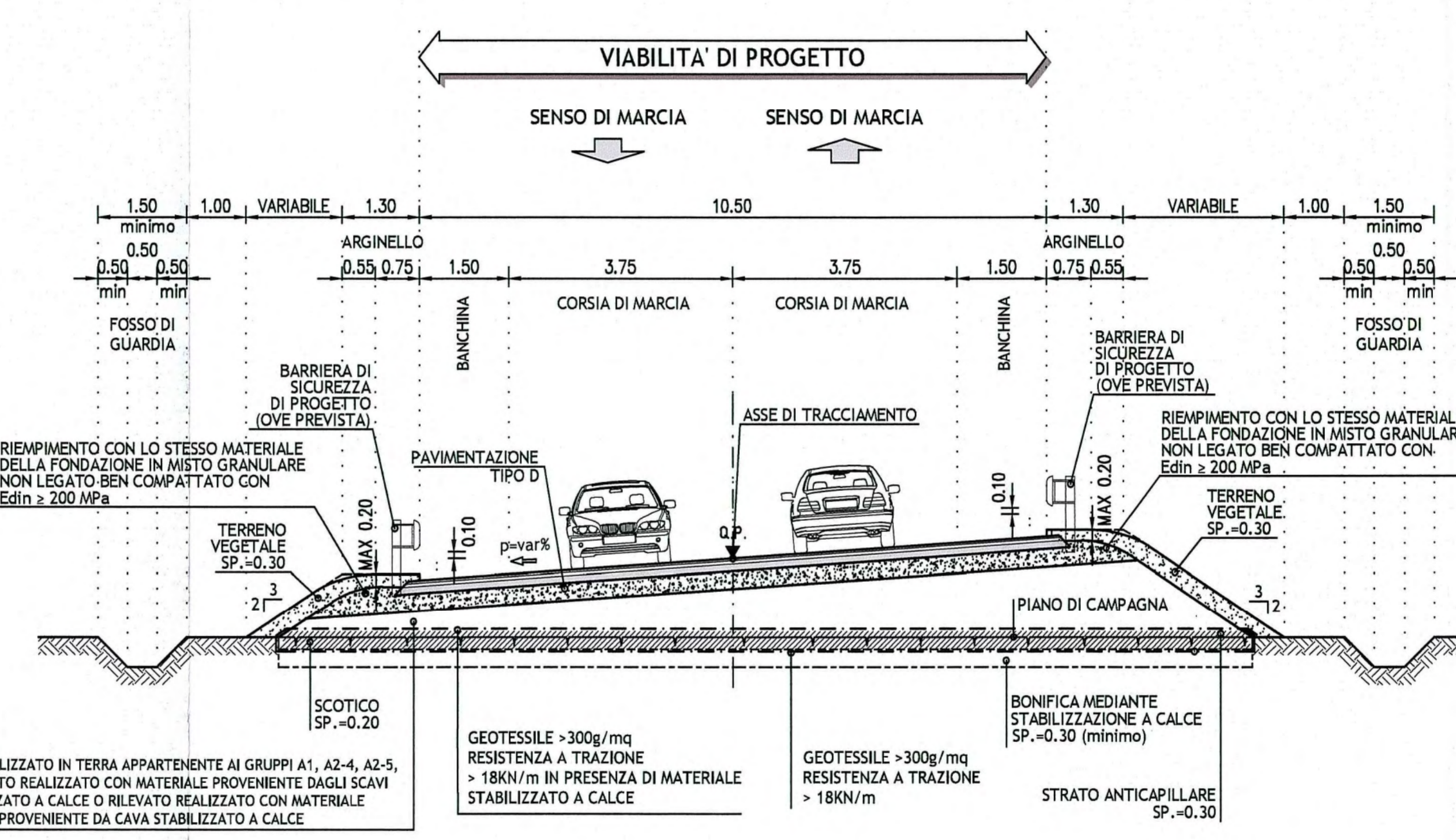
Tipo 1b in curva VIABILITA' INTERFERENTE IN CURVA CON RILEVATO H < 5.50m - scala 1:100 CATEGORIA "C1" (DM 05/11/2001) STRADE EXTRAURBANE SECONDARIE
