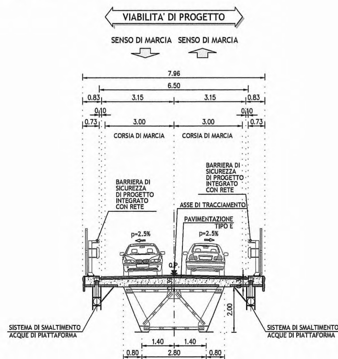
Tipo 2 su cavalcavia IN RETTILINEO - scala 1:100 SEZIONE TIPO IN CAMPATA CAVALCAVIA "CA.06"
