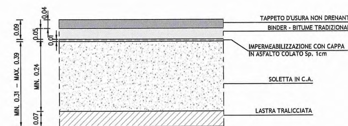
Pacchetto su opera d'arte scala 1:10 PAVIMENTAZIONE TIPO "E" - CAVALCAVIA "CA.06"
