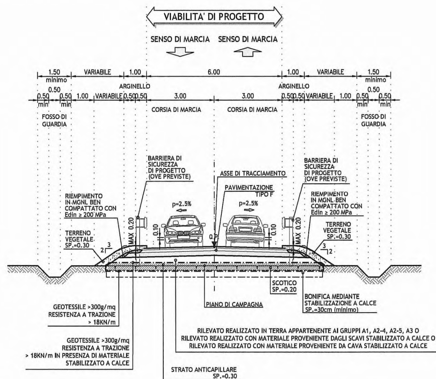
Tipo 1a in rilevato IN RETTILINEO - scala 1:100 STRADE LOCALI A DESTINAZIONE PARTICOLARE
