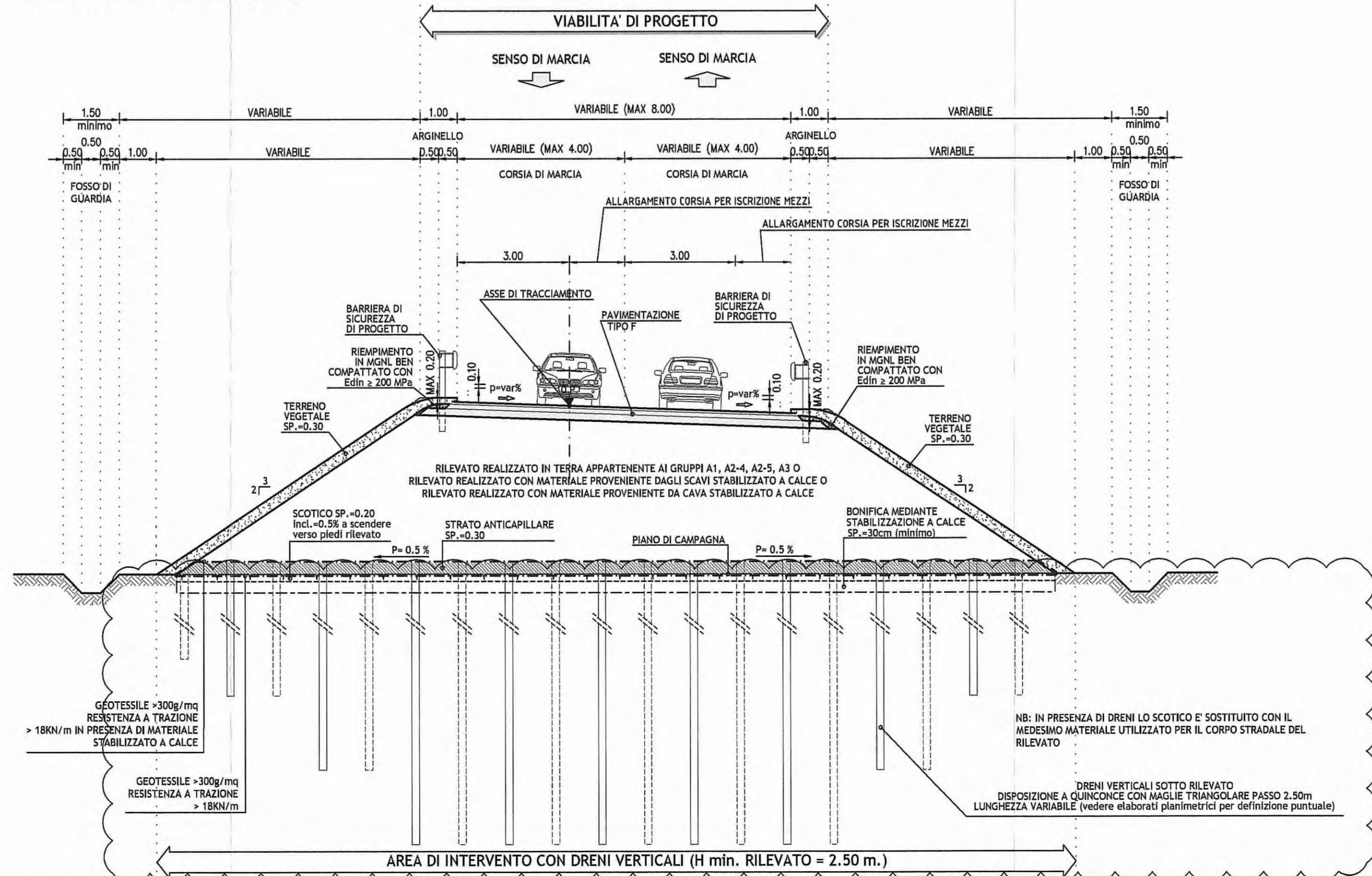
Tipo 1c in rilevato IN CURVA CON ALLARGAMENTO PER ISCRIZIONE MEZZI (CON PRESENZA DI DRENI) - scala 1:100 STRADE LOCALI A DESTINAZIONE PARTICOLARE
