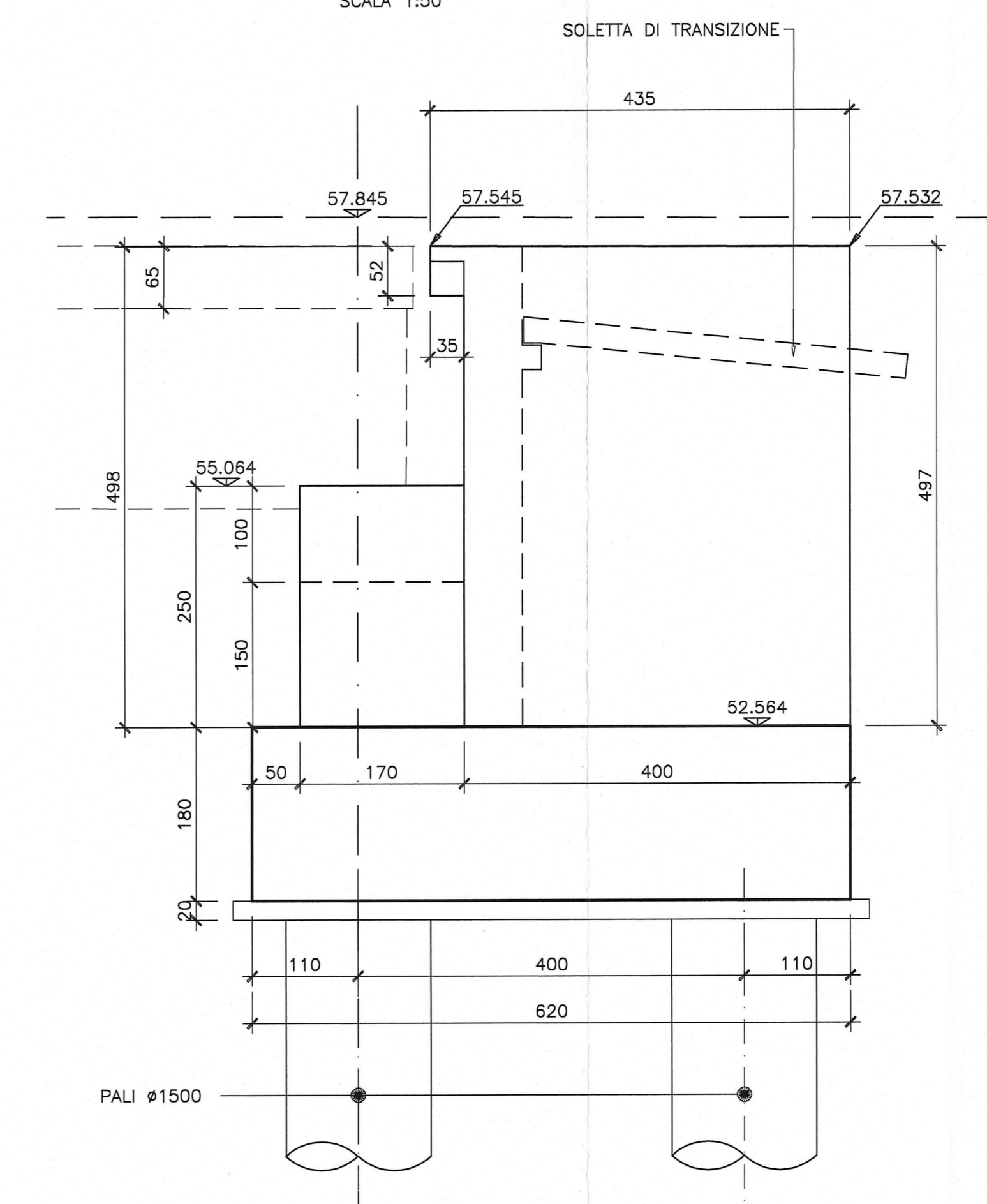
VISTA C SCALA 1:50
