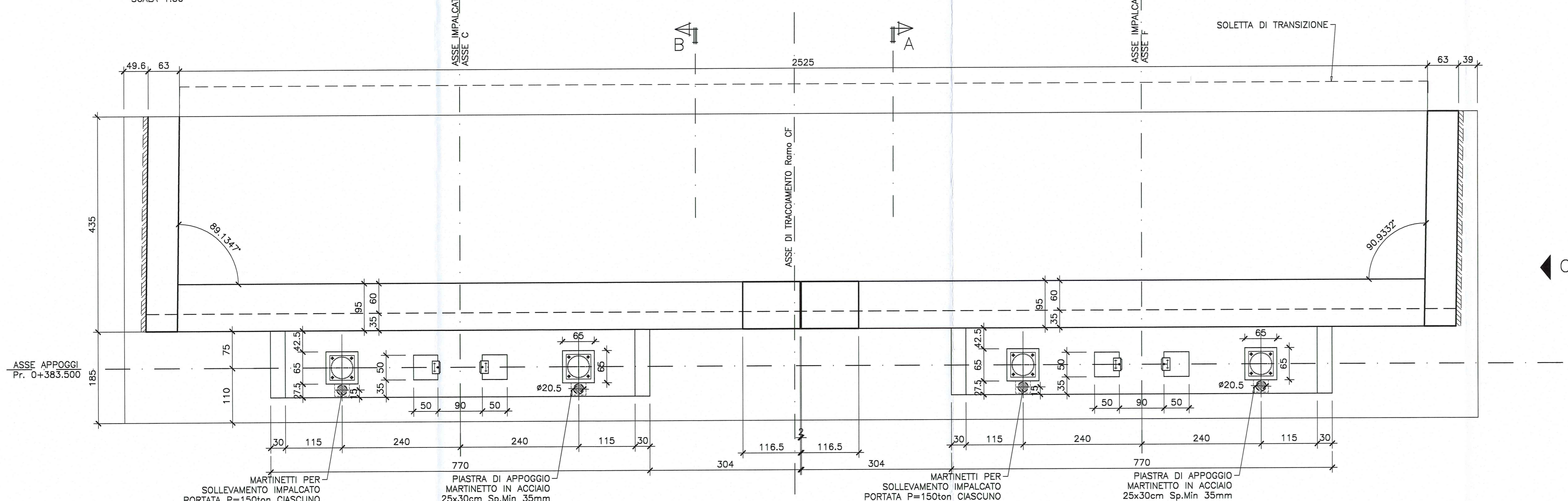
PIANTA VISTA DALL'ALTO SCALA 1:50
