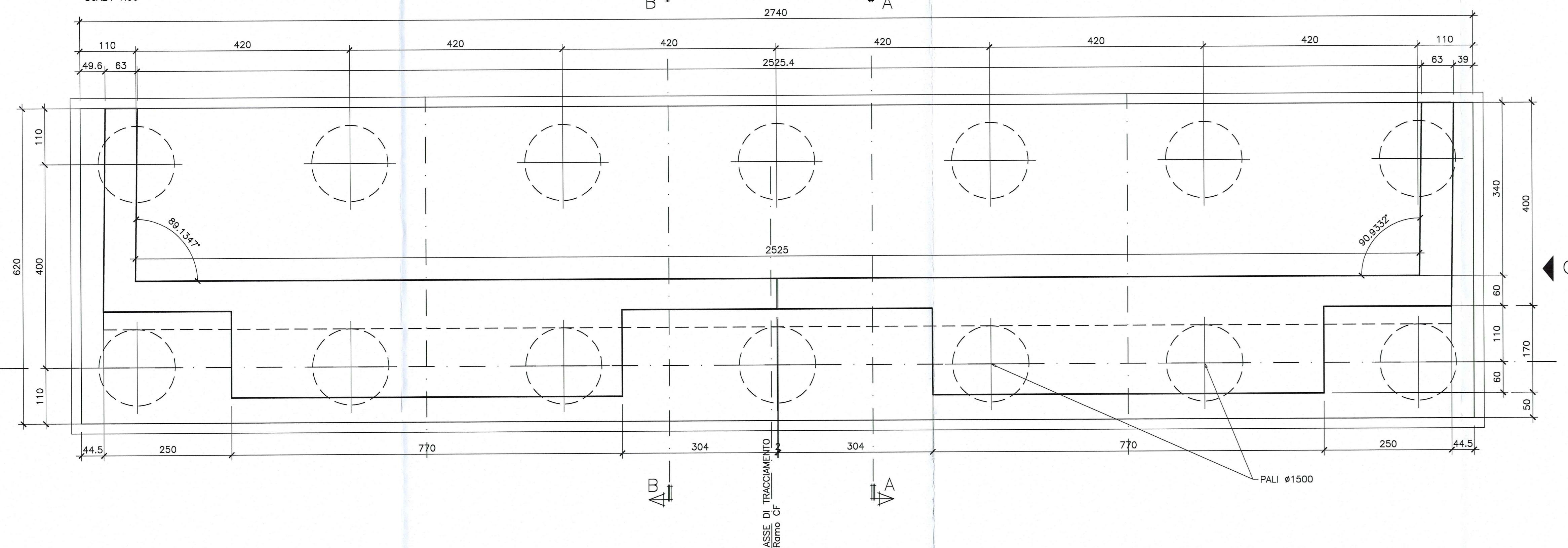
PIANTA FONDAZIONI E SPICCATI SCALA 1:50
