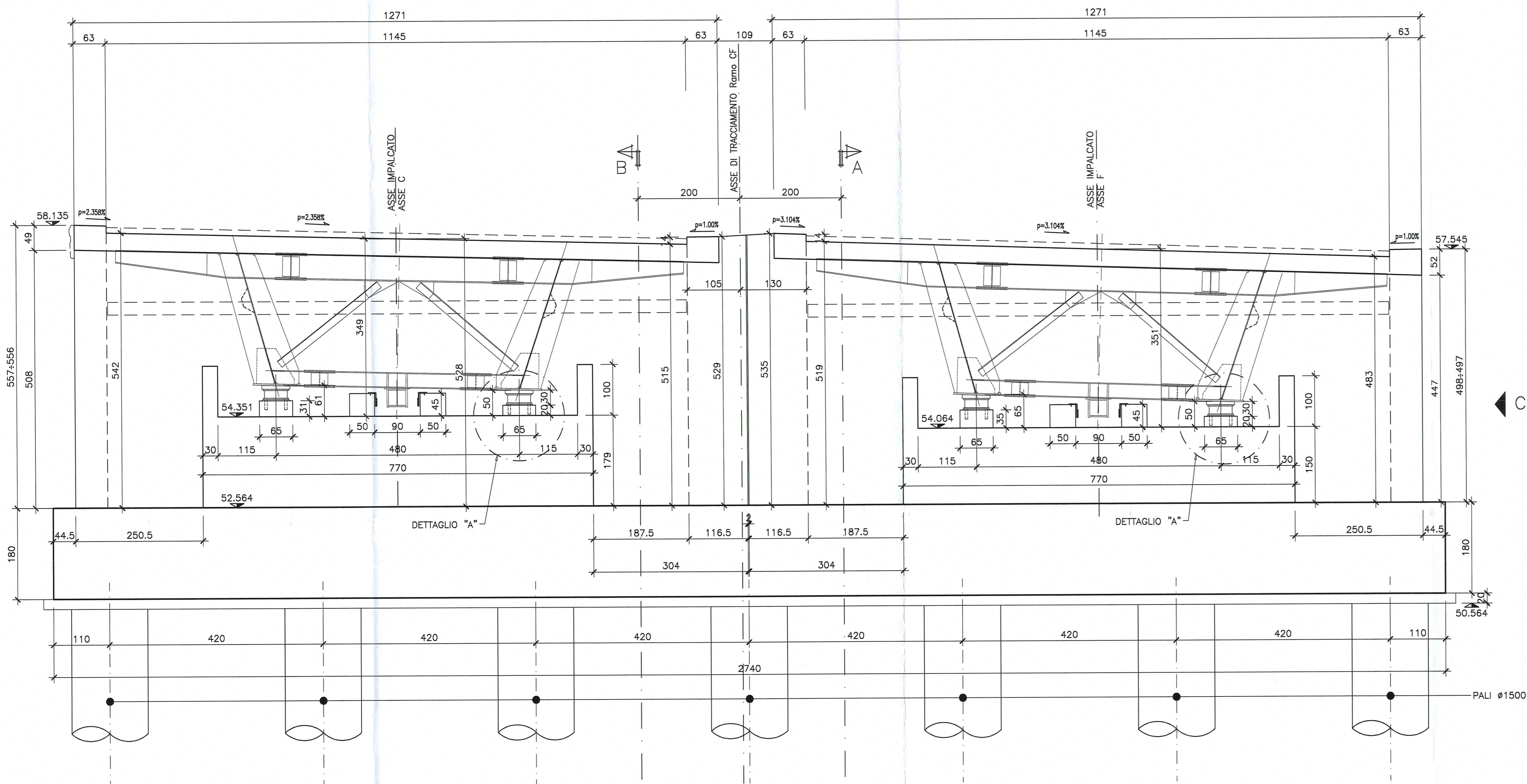
VISTA FRONTALE SCALA 1:50
