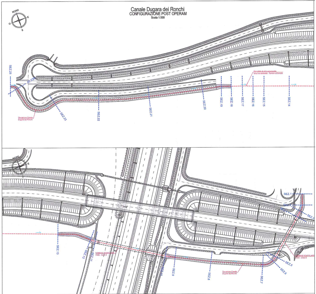
Canale Dugara dei Ronchi – planimetria sezioni di studio Post Operam
