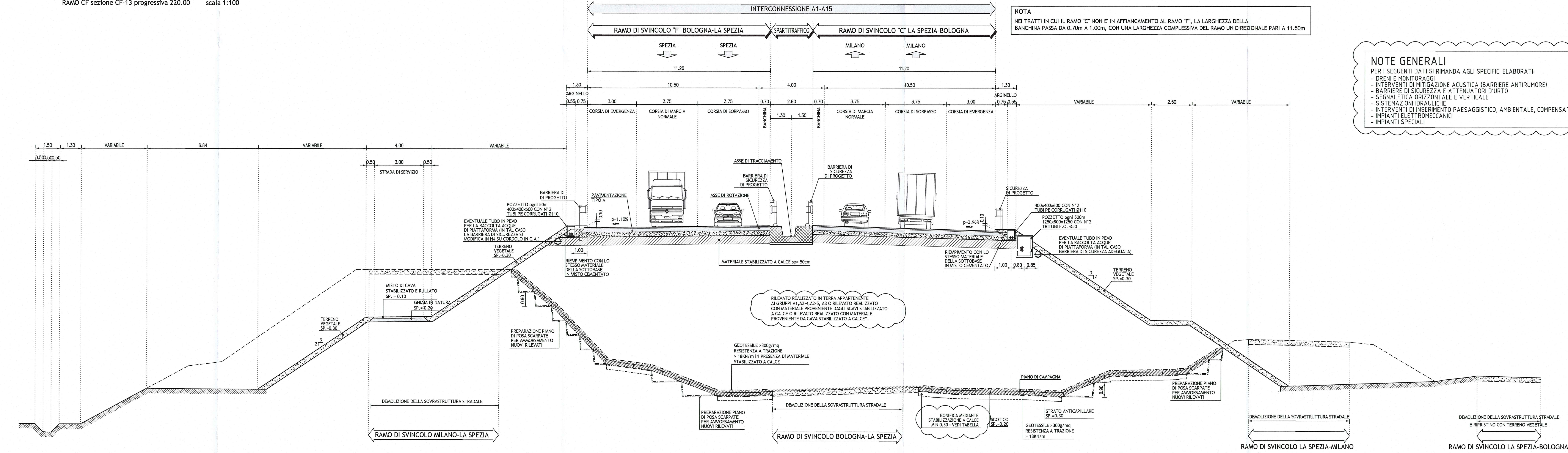
Tipo 1n in rilevato VIABILITA' RAMO DI SVINCOLO BIDIREZIONALE A DUE CORSIE RAMO CF sezione CF-13 progressiva 220.00 scala 1:100
