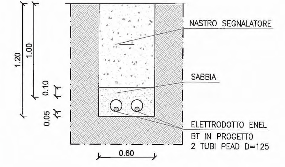
SEZIONE TIPO 2 TUBI PEAD D=125 - BASSATENSIONE SCALA 1:25
