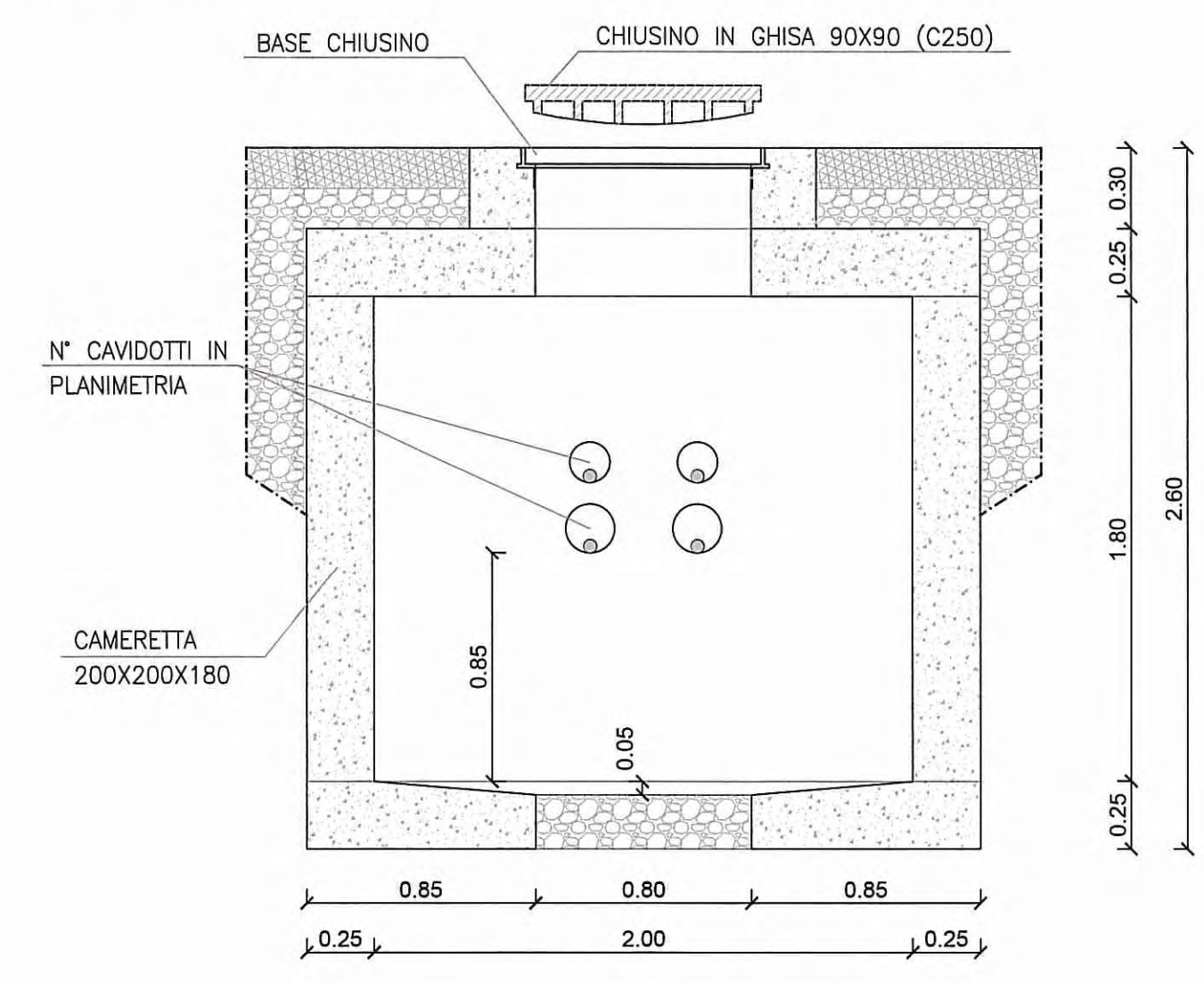
CAMERETTA TIPO DA 200x200x180 h SCALA 1:25
