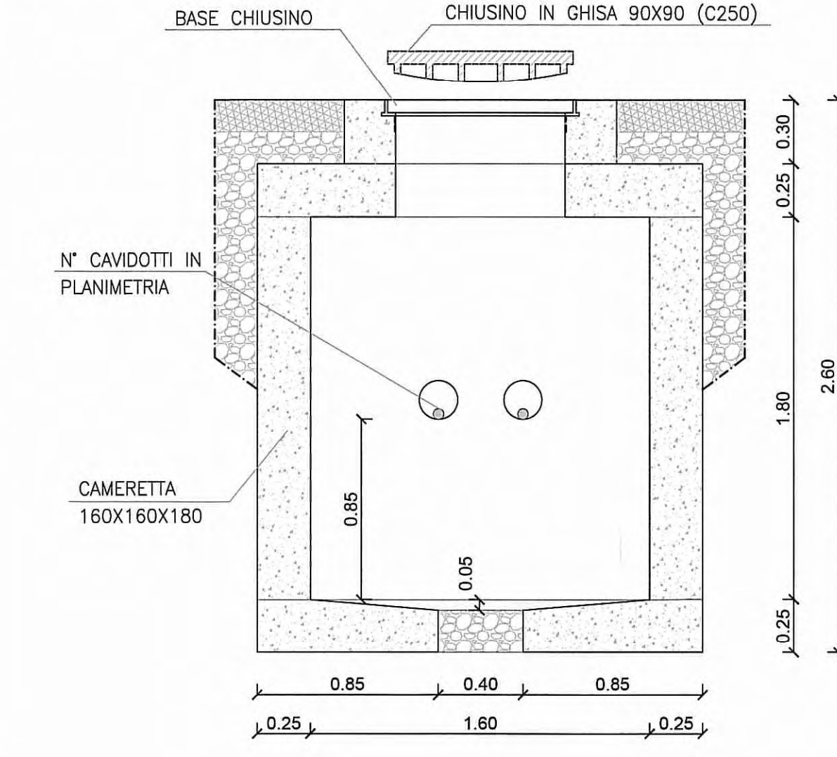
CAMERETTA TIPO DA 160x160x180 h SCALA 1:25
