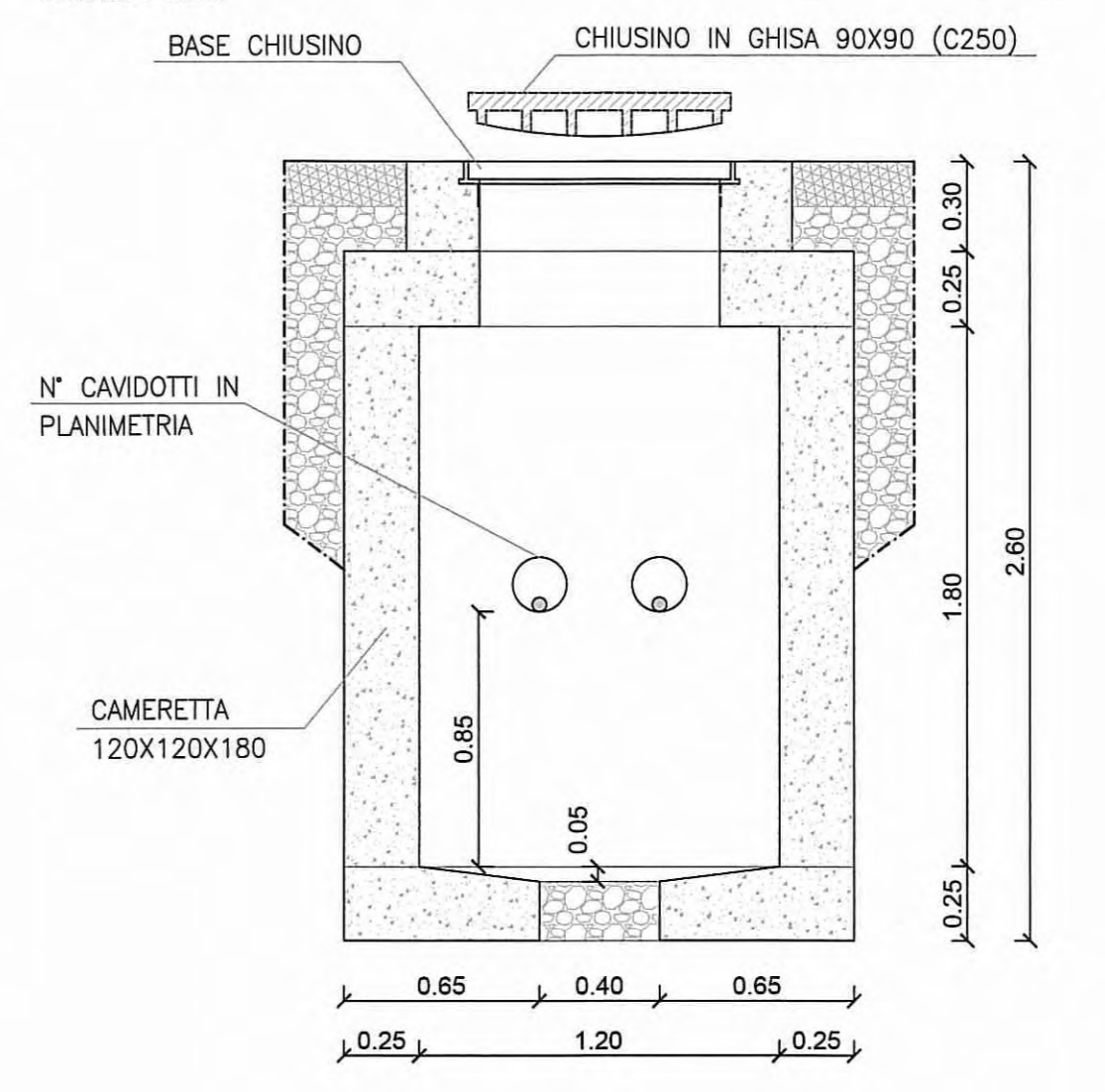
CAMERETTA TIPO DA 120x120x180 h SCALA 1:25
