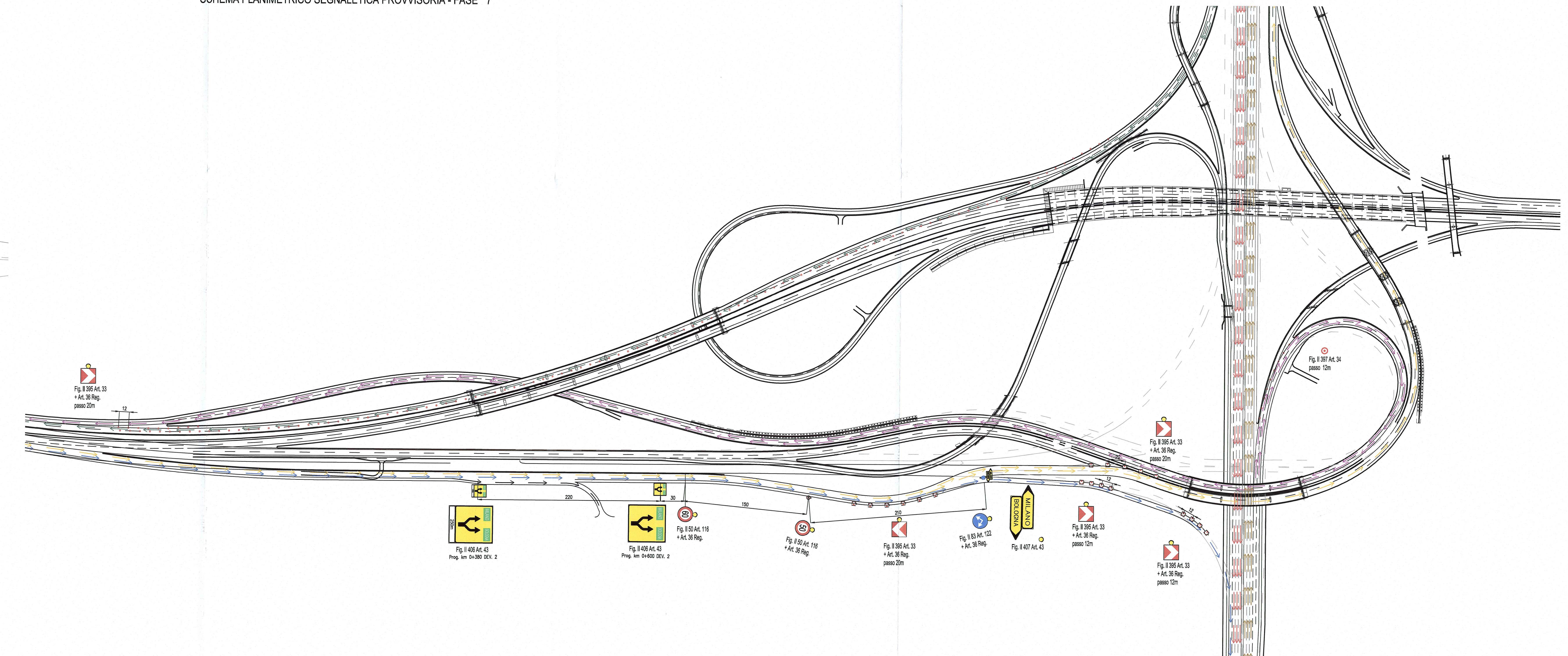
SCHEMA PLANIMETRICO SEGNALETICA PROVVISORIA - FASE "7"
