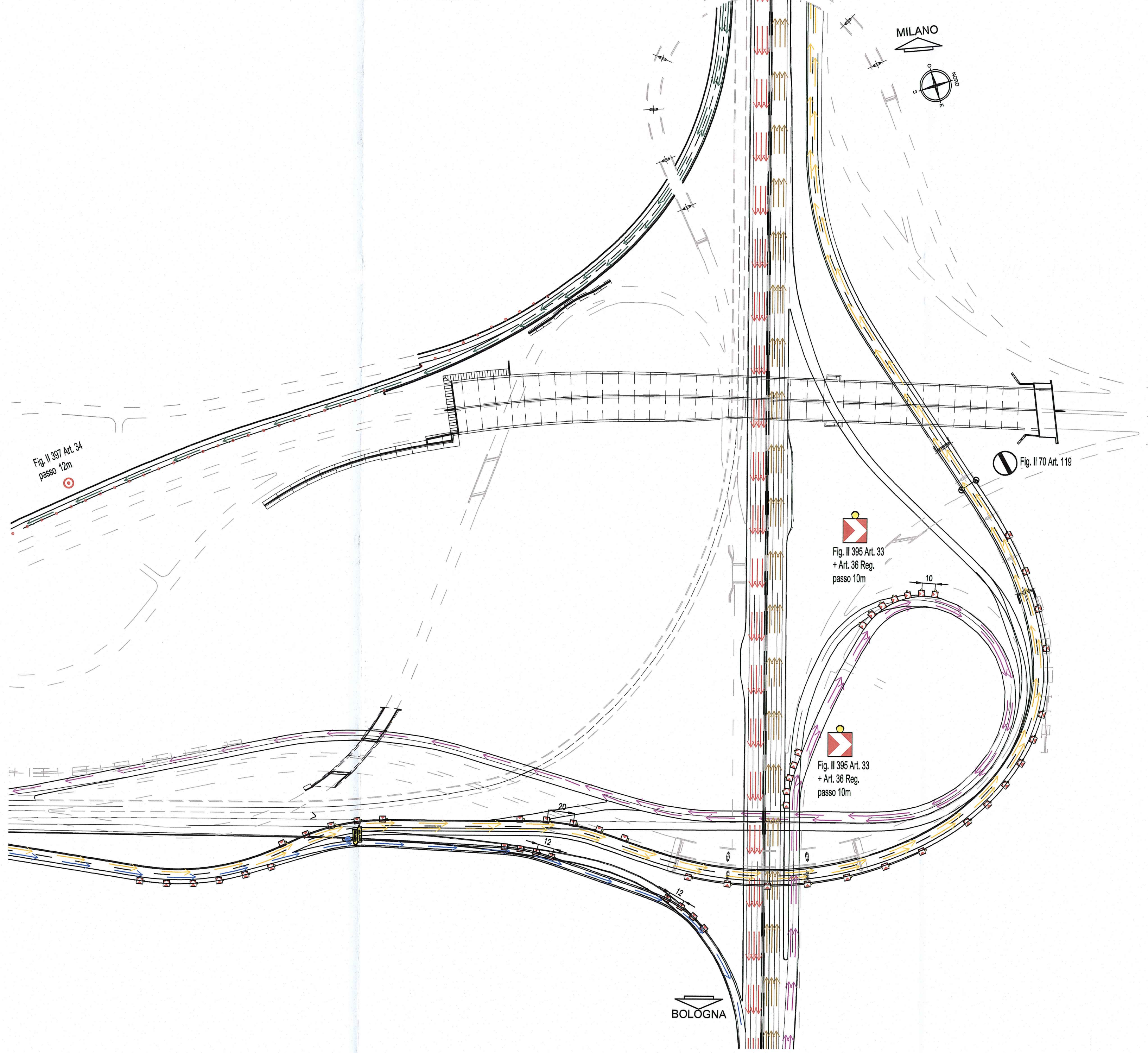
SCHEMA PLANIMETRICO SEGNALETICA PROVVISORIA - FASE "5"
