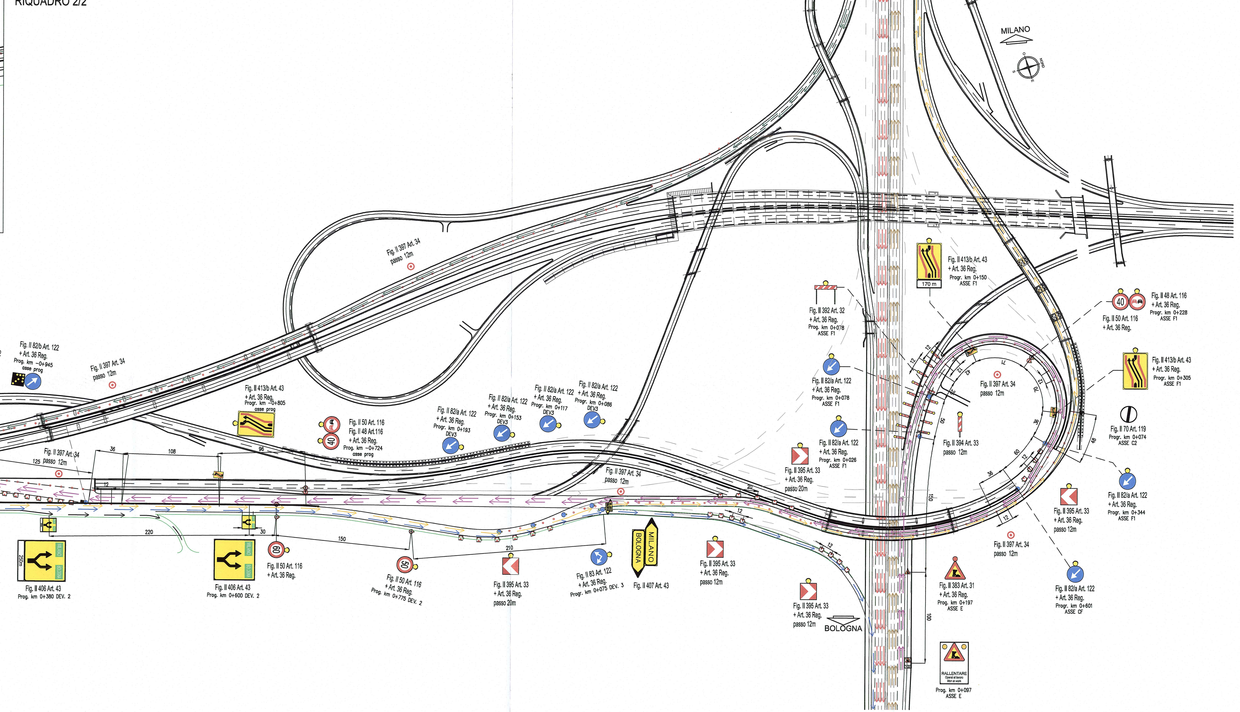
SCHEMA PLANIMETRICO SEGNALETICA PROVVISORIA - FASE "6" RIQUADRO 2/2
