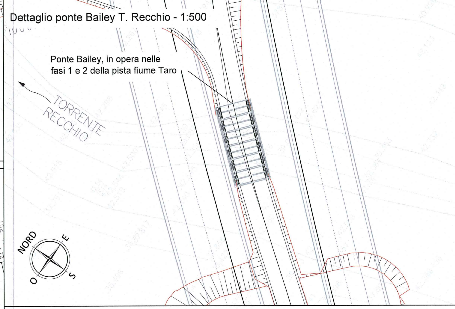
Dettaglio ponte Bailey T. Recchio - 1:500
