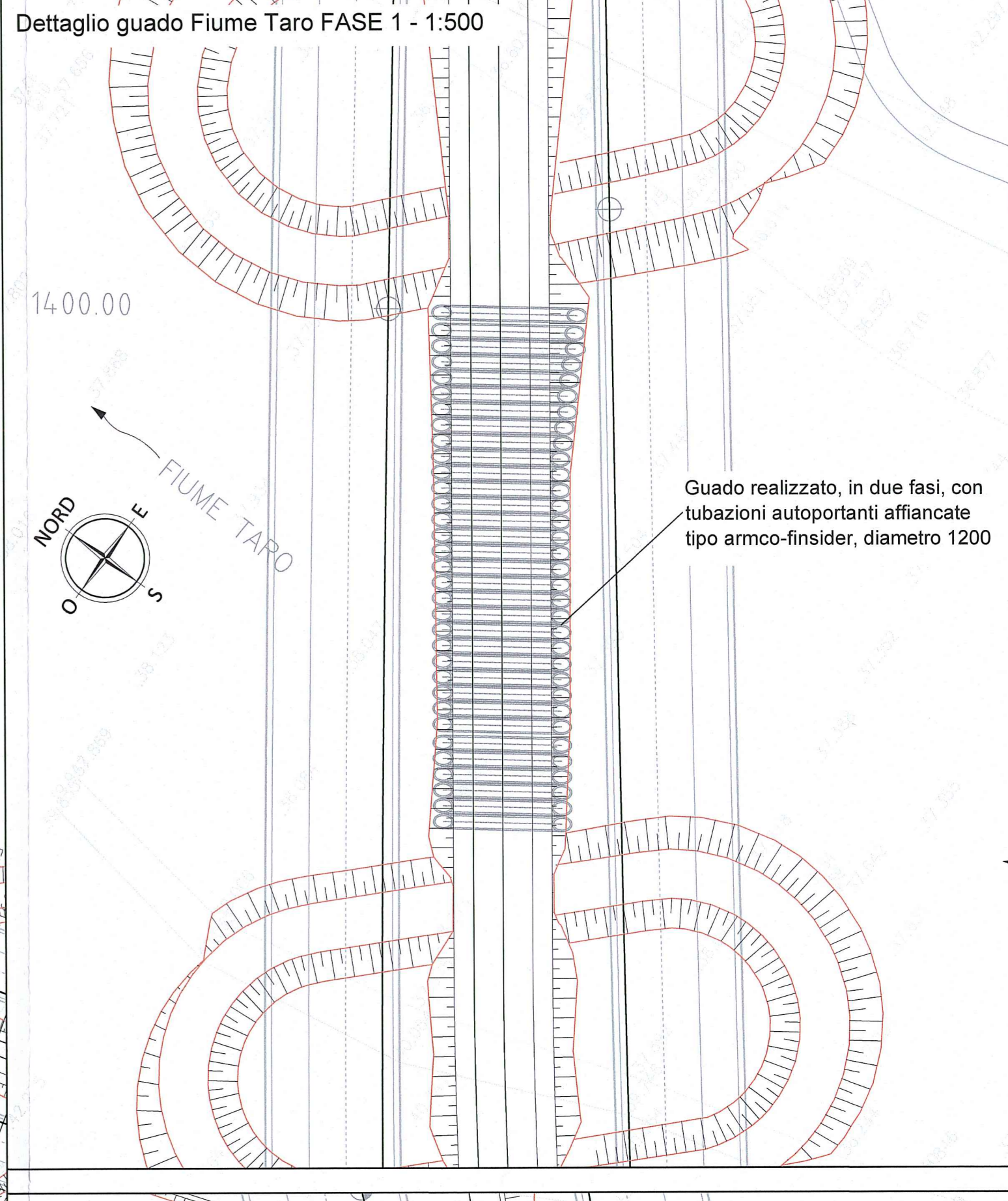
1 Planimetria di progetto - 1:1000
