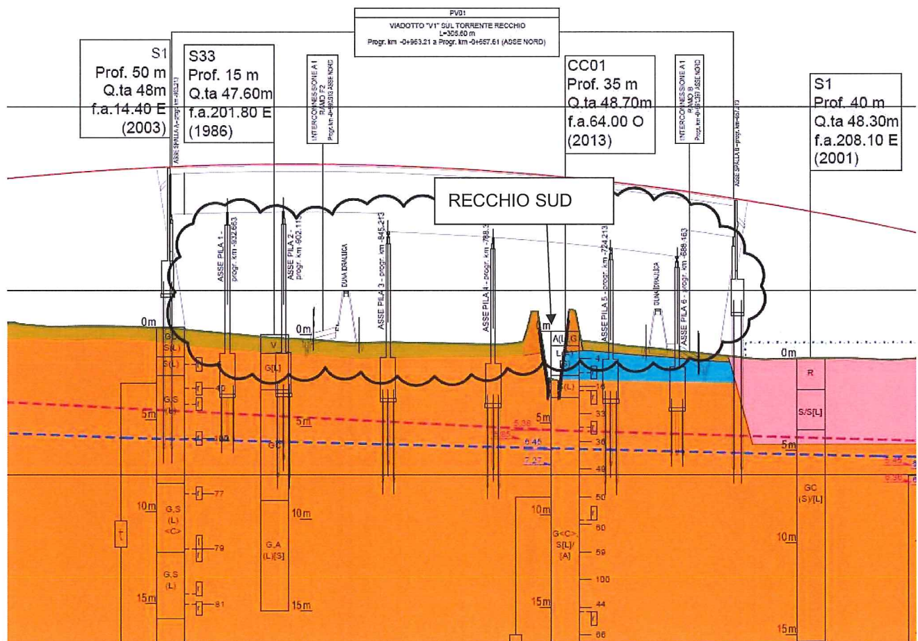
Figura 1: Estratto profilo geotecnico
