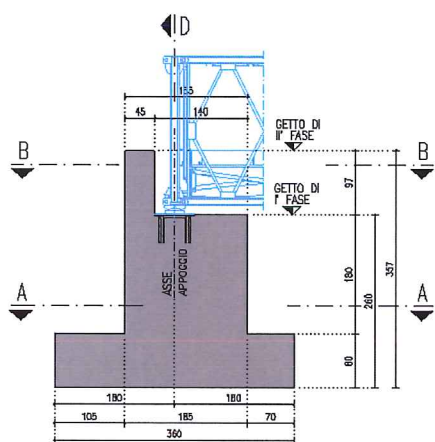
SEZIONE LONGITUDINALE C-C scala 1:50
