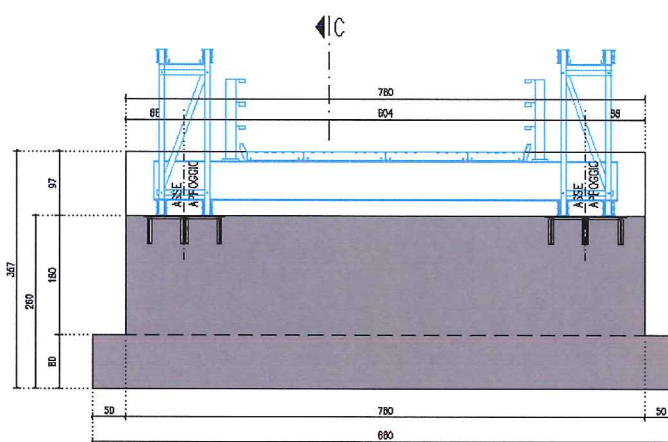
SEZIONE TRASVERSALE D-D scala 1:50
