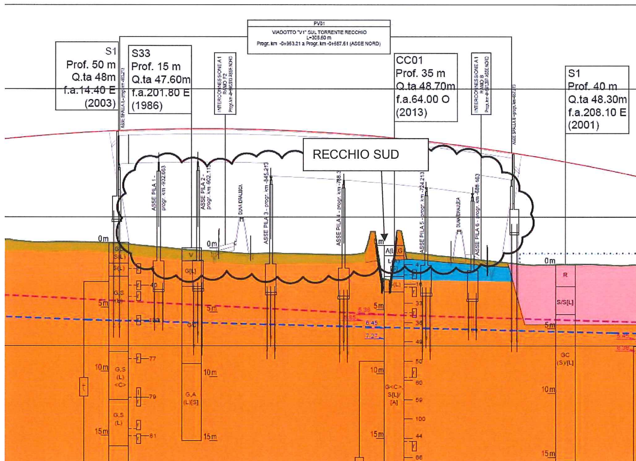
Figura 1: Estratto profilo geotecnico
