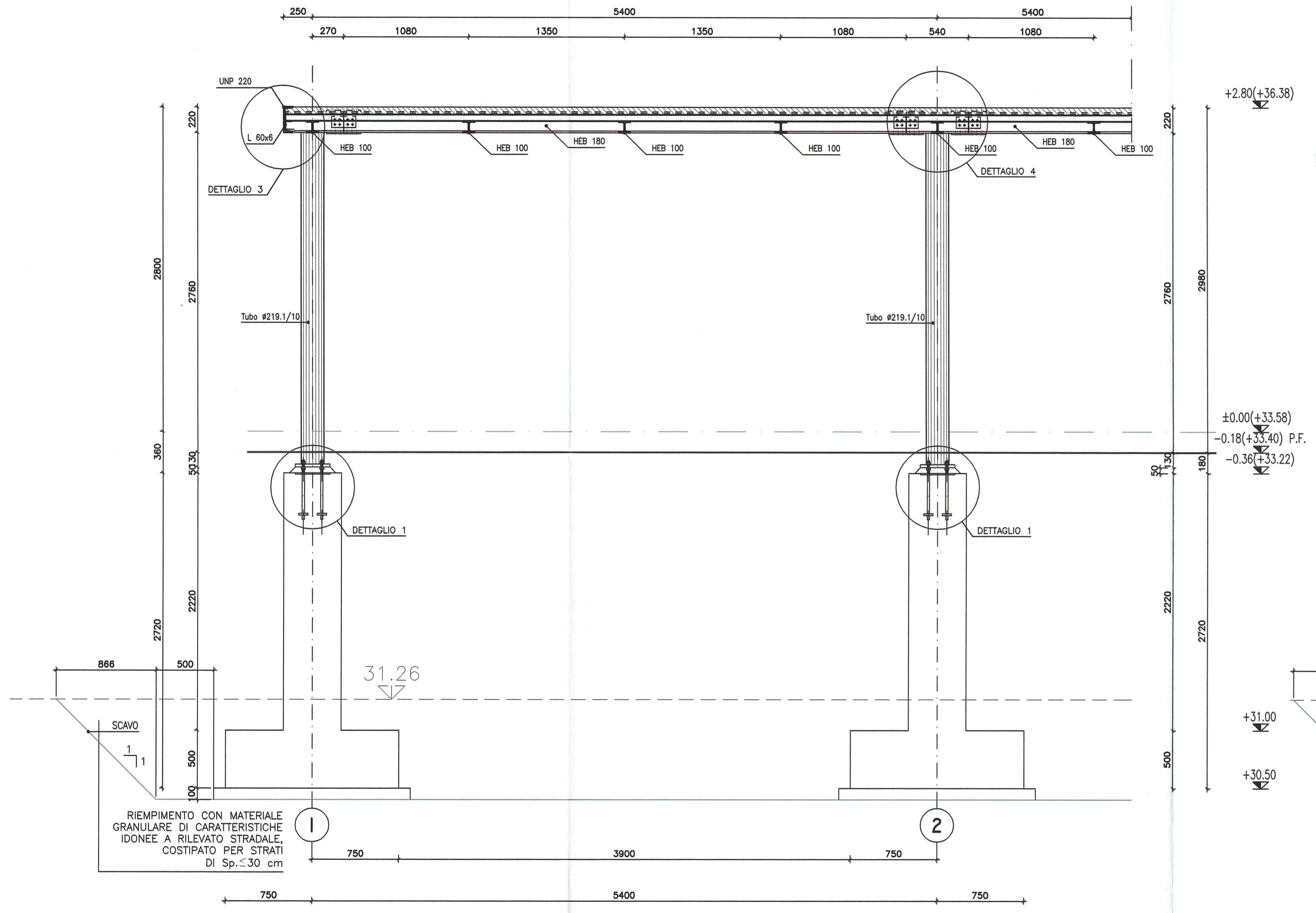
SEZIONE A-A SCALA 1:25
