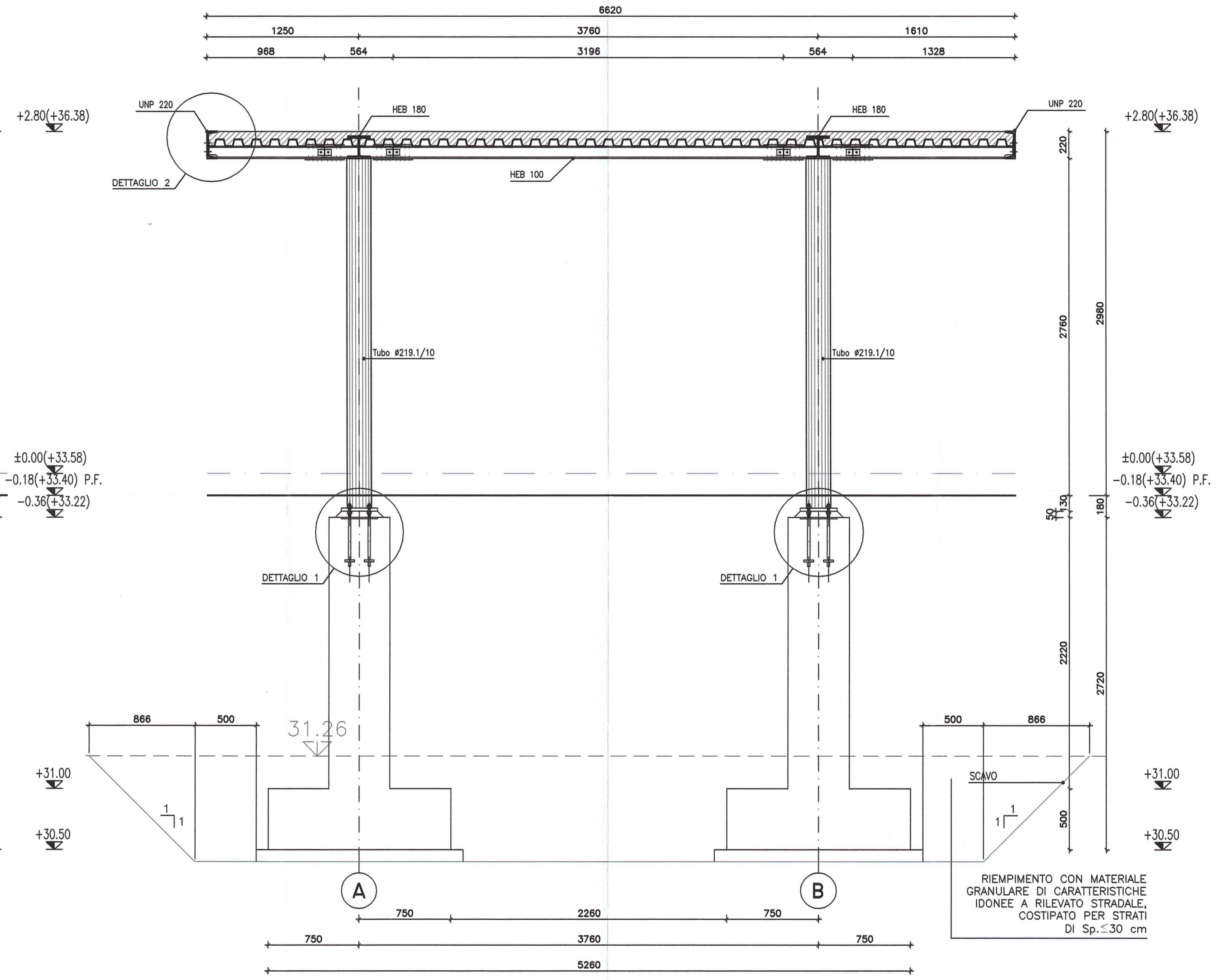
SEZIONE B-B SCALA 1:25
