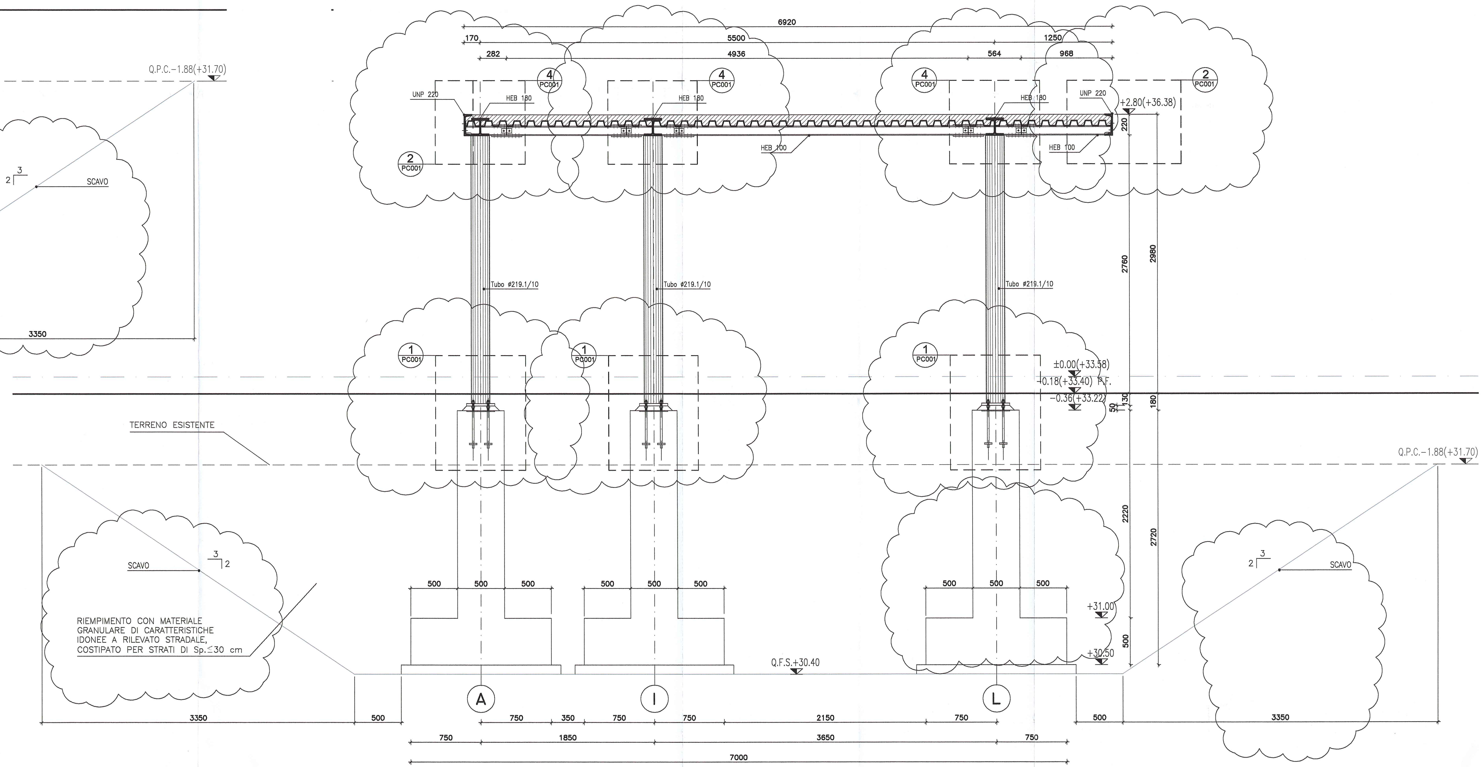
SEZIONE B-B SCALA 1:25
