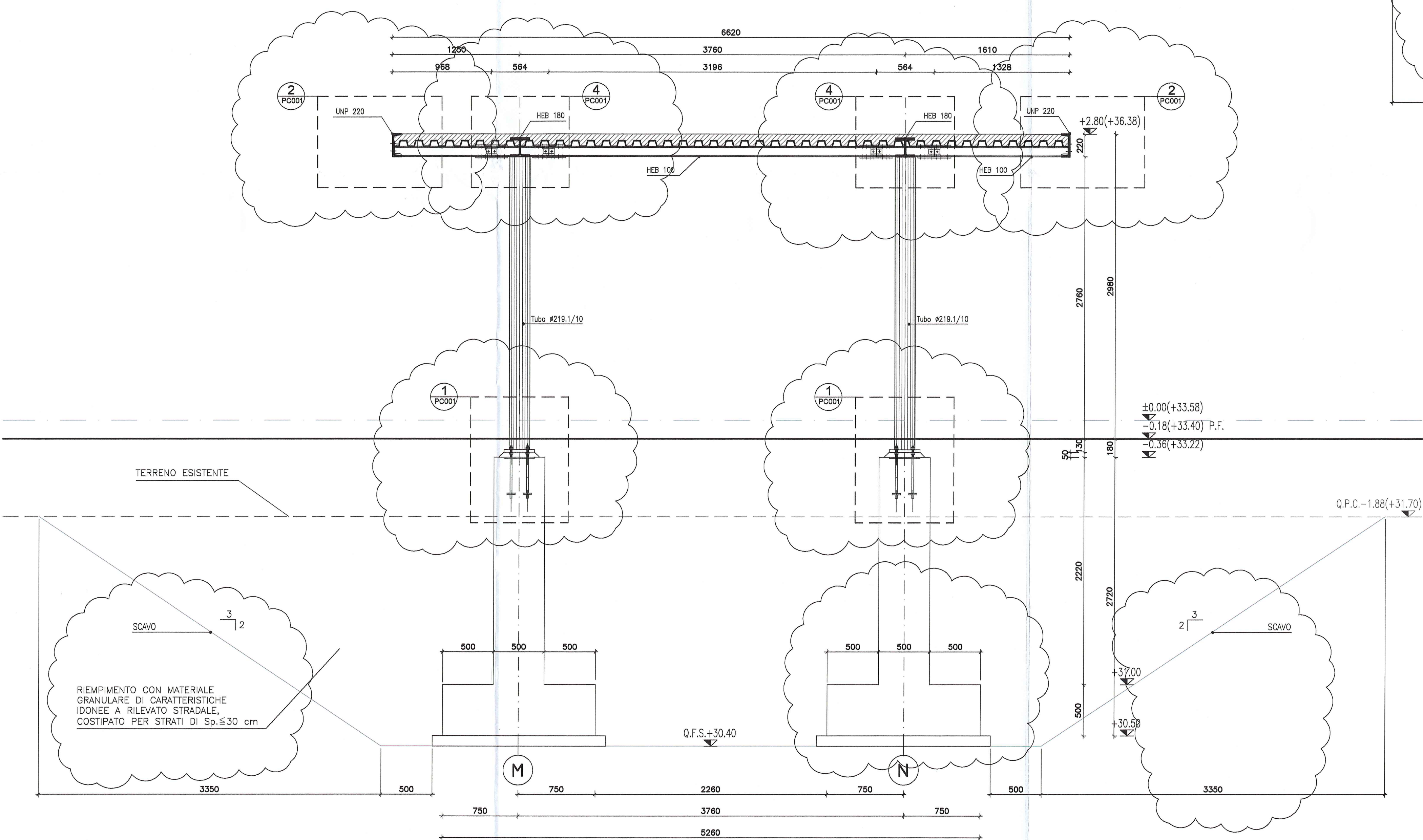
SEZIONE C-C SCALA 1:25
