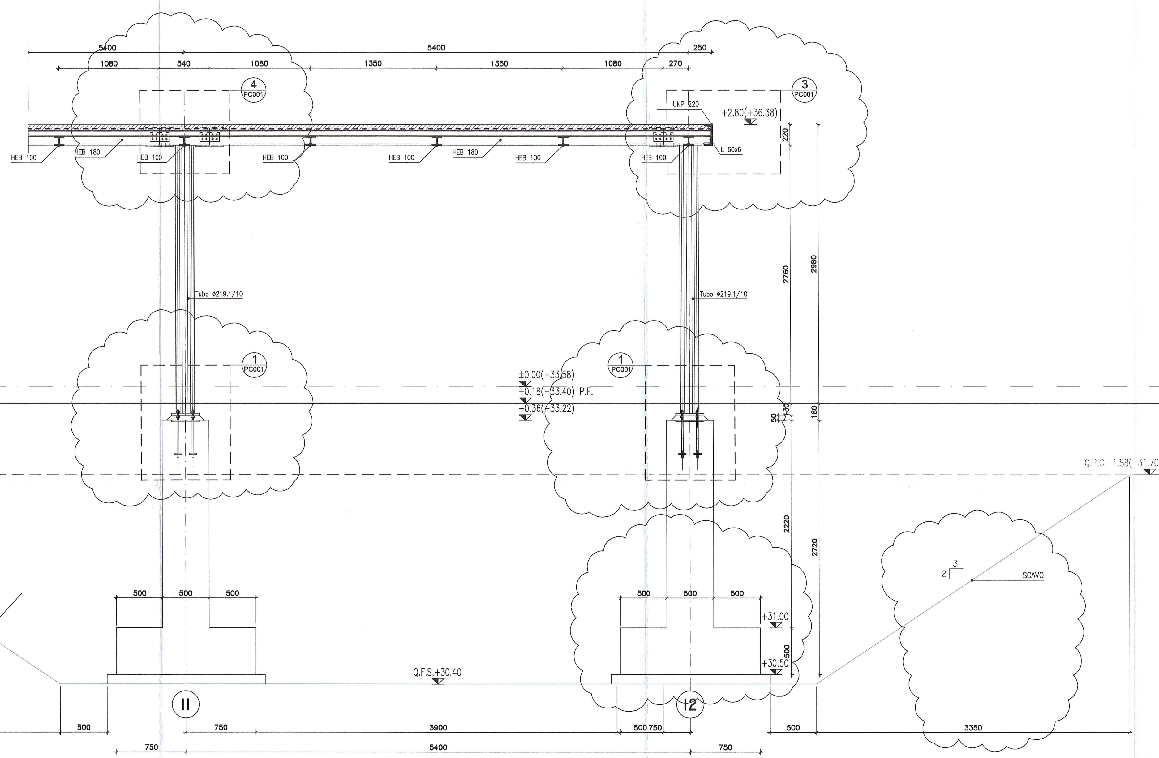
SEZIONE A-A SCALA 1:25
