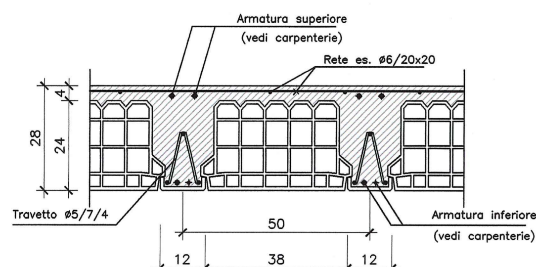
SEZIONE SOLAIO TIPICO SCALA 1:10
