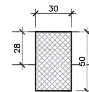
SEZIONE TIPO T3 (30x50) Scala 1:20
