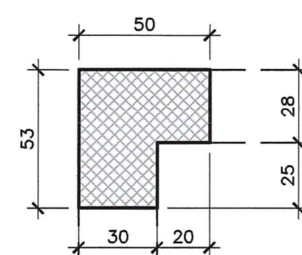
SEZIONE TIPO T1 Scala 1:20
