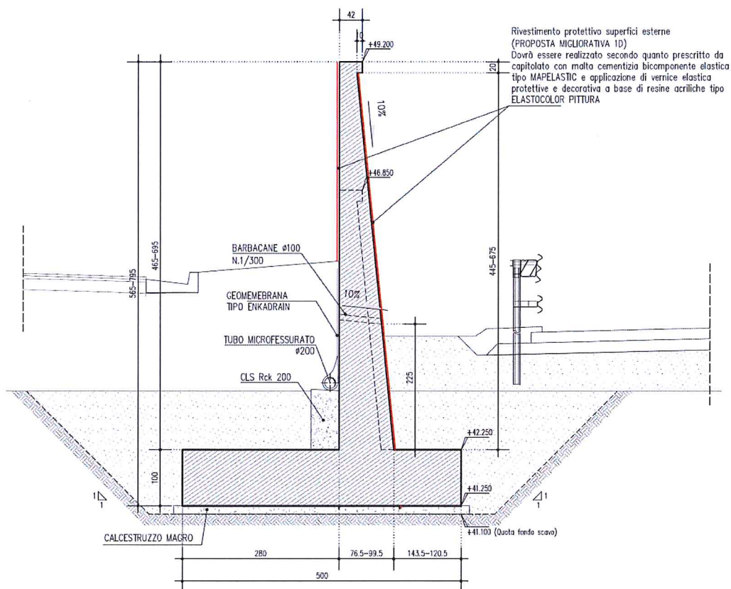
Figura 1-2 – Concio 1 e 2
