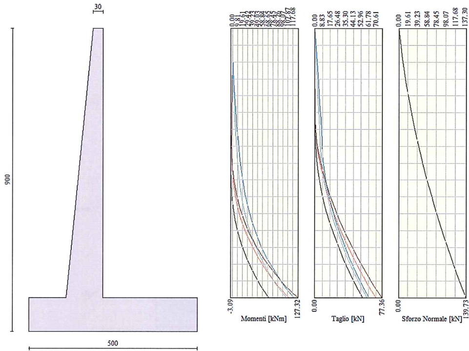
Figura 12-3 – Involuppo sollecitazioni SLE
