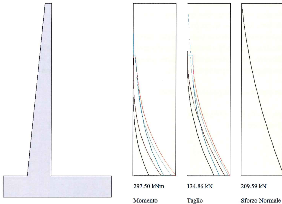
Figura 12-1 – Inviluppo sollecitazioni SLU-STATICA
