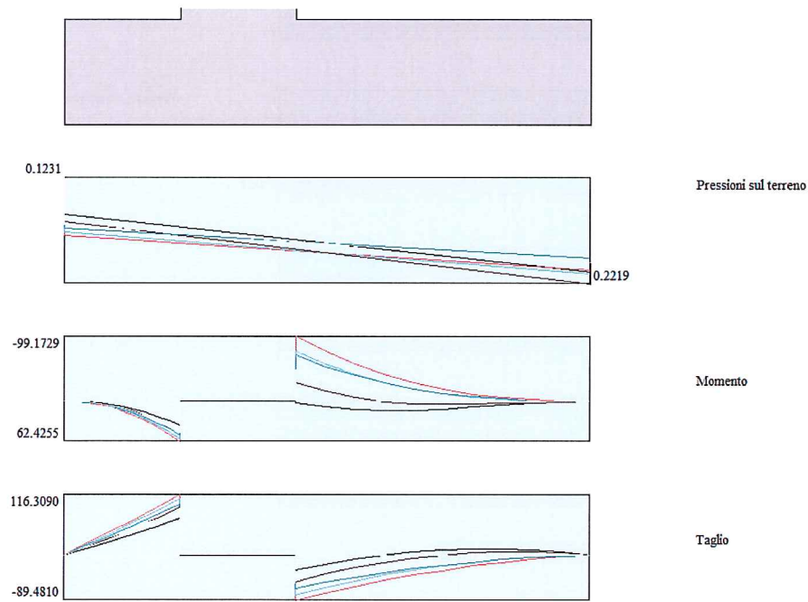
Figura 12-4 – Involuppo sollecitazioni SLU-STATICA
