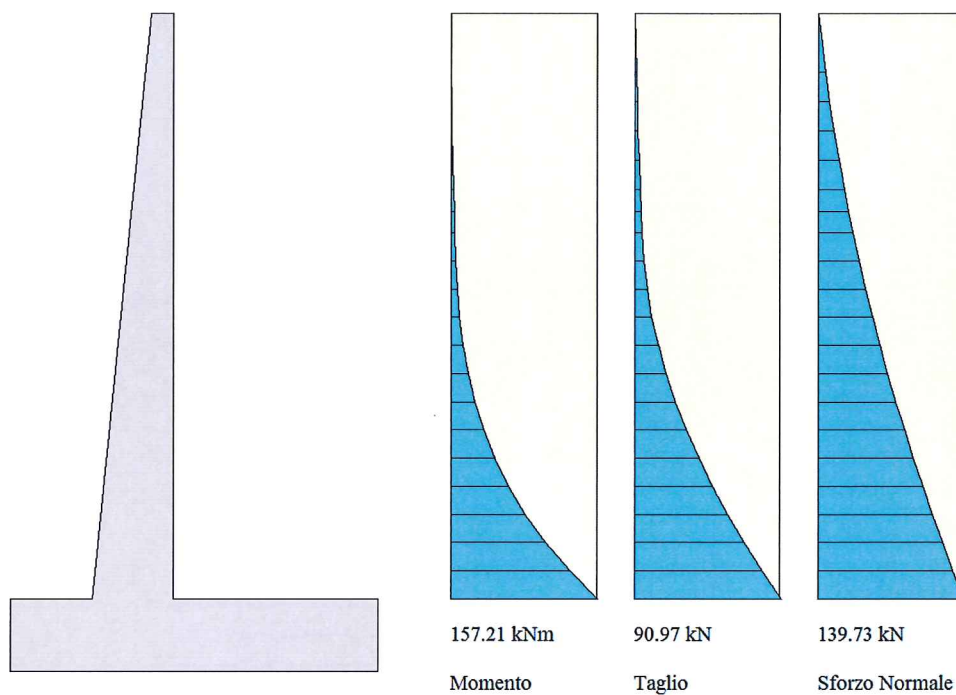
Figura 12-2 – Sollecitazioni SLU-SISMICA
