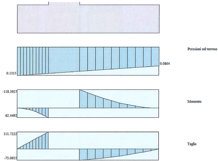
Figura 12-5 – Sollecitazioni SLU-SISMICA
