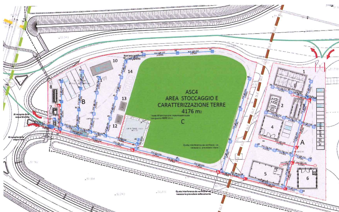
Figura 1 – Lay-out delle reti fognarie a servizio dell'area di cantiere in esame.
