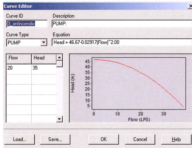
Punti caratteristici di funzionamento delle pompe dell'impianto di pressurizzazione del cantiere PV
