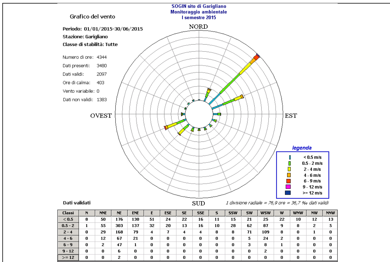
Figura 3-2 Rosa dei venti – I° semestre 2015
