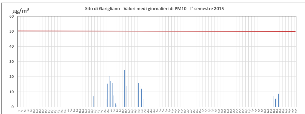
Figura 3-5 PM10 - Andamenti dei valori medi giornalieri - Cantiere I° semestre 2015
