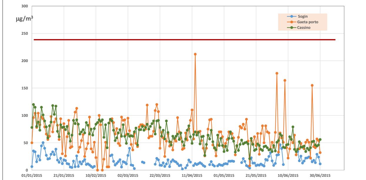
Figura 3-4 NO 2 – III Campagna in corso d'opera - Confronto con i dati delle centraline ARPA Lazio - Andamenti dei valori massimi orari sull'intero periodo di monitoraggio
