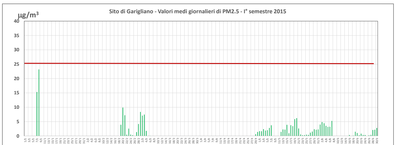
Figura 3-7 PM2.5 - Andamenti dei valori medi giornalieri - Cantiere I° semestre 2015
