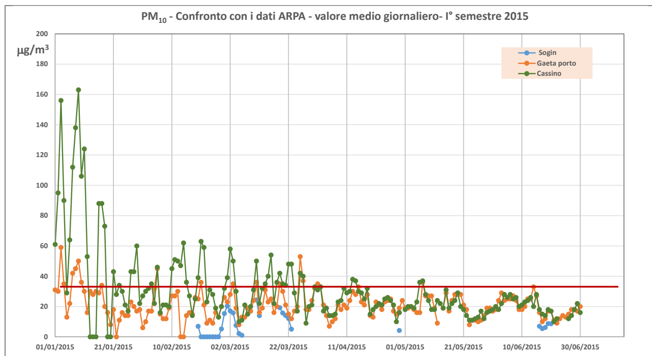
Figura 3-6 PM 10 – Confronto con i dati delle centraline ARPA Lazio
