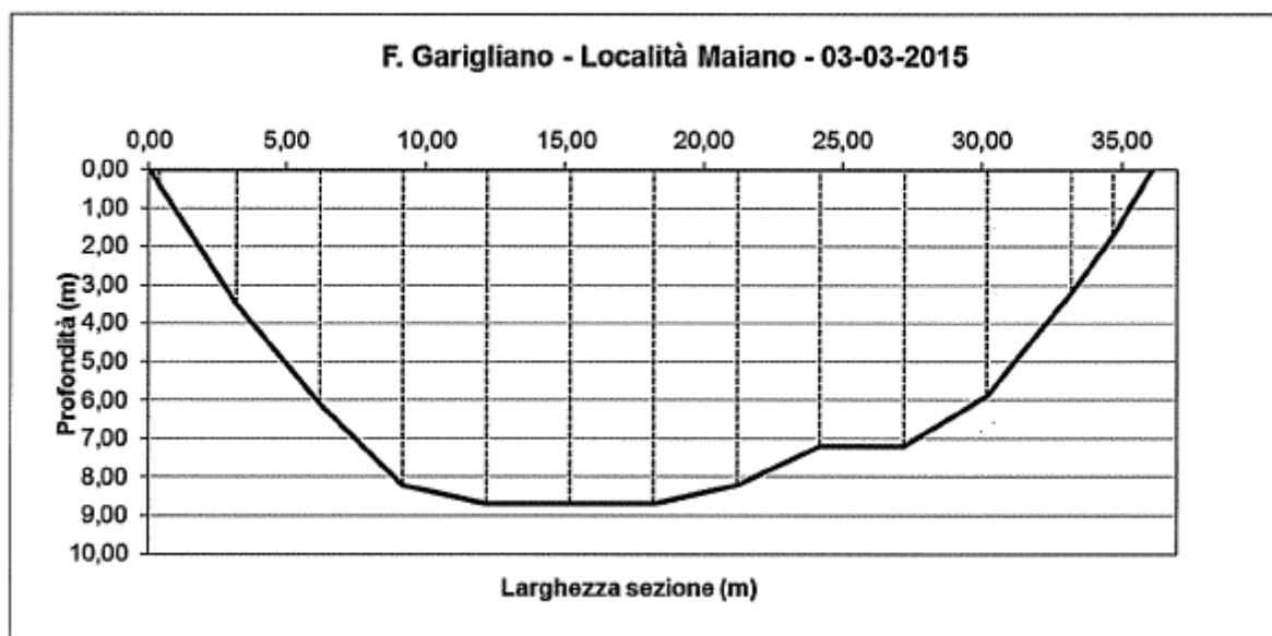
Figura 4-1 - Profilo della sezione di misura
