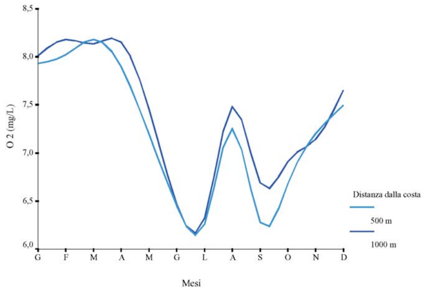
ANDAMENTO DELLE MEDIE MENSILI A 500 m E A 1000 m COSTA TIRRENICA
