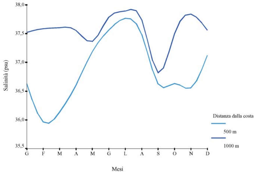
SALINITA': ANDAMENTO DELLE MEDIE MENSILI A 500 m E A 1000 m COSTA TIRRENICA
