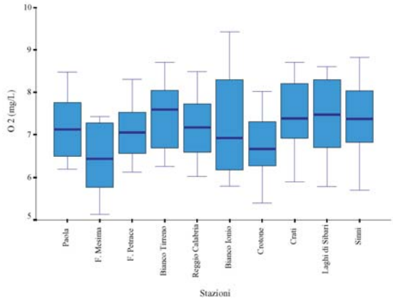
RAPPRESENTAZIONE DELLE DISTRIBUZIONI DEI DATI A 500 m
