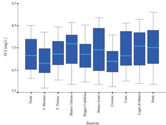
RAPPRESENTAZIONE DELLE DISTRIBUZIONI DEI DATI A 1000 m
