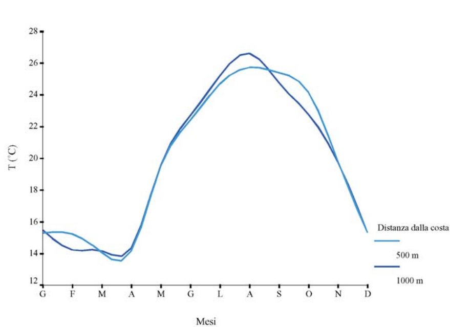
TEMPERATURA: ANDAMENTO DELLE MEDIE MENSILI A 500 m E A 1000 m COSTA TIRRENICA
