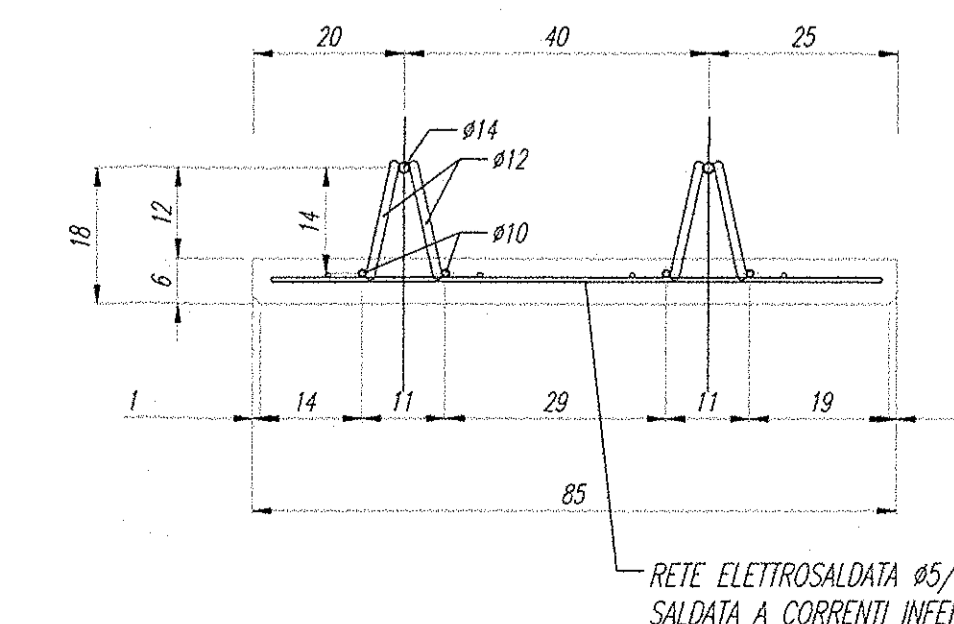
SEZIONE TRASVERSALE LASTRE TIPO D, D1, D2, J1, J2 SCALA 1:10
