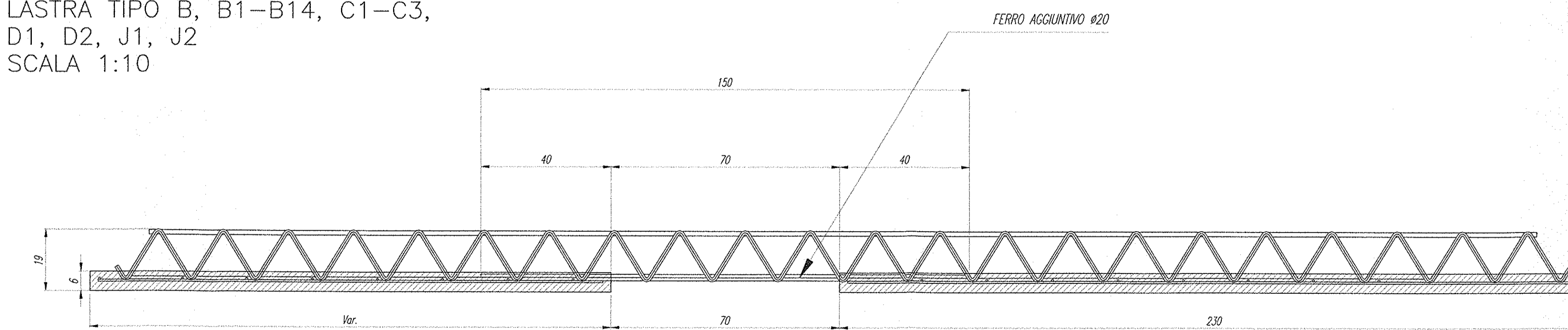
SEZIONE TRASVERSALE LASTRE TIPO B, B1-B14, C1-C3 SCALA 1:10
