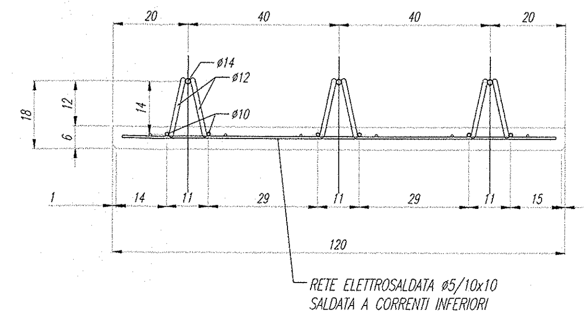
SEZIONE TRASVERSALE LASTRE TIPO B, B1-B14, C1-C3 SCALA 1:10
