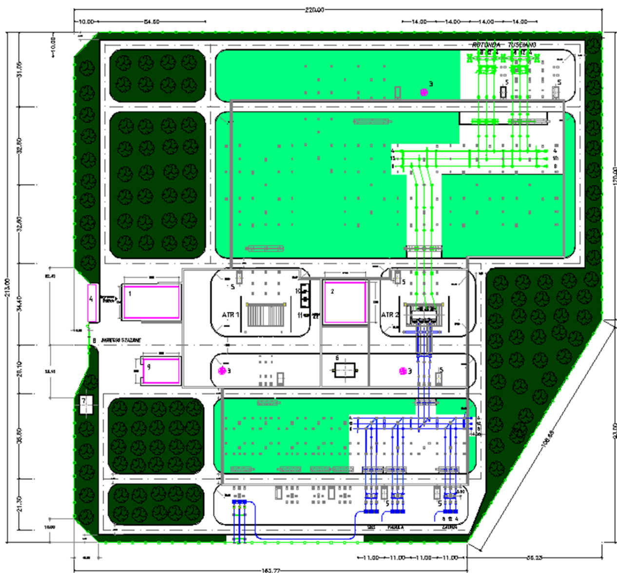
Figura 1 – Planimetria generale della stazione 220/150 kV: in grigio la precedente soluzione progettuale, in verde e blu la nuova configurazione di progetto che prevede la realizzazione del solo “ATR2”. Lo stato atteso a fine intervento è riportato nella planimetria di progetto della stazione (dis. DUFR10014BER10011).
