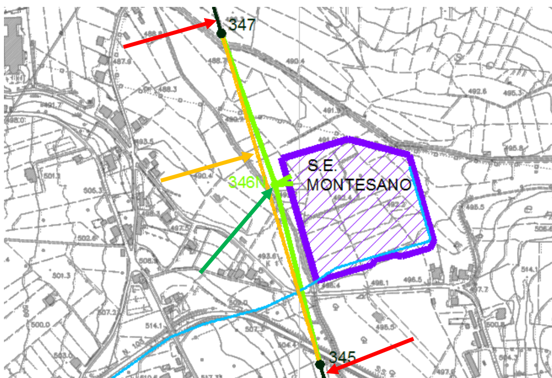
Figura 2 – Opere previste. Le frecce rosse indicano la linea esistente, la freccia arancio indica il tratto da demolire, la freccia verde indica il nuovo sostegno in doppia terna previsto dal progetto
