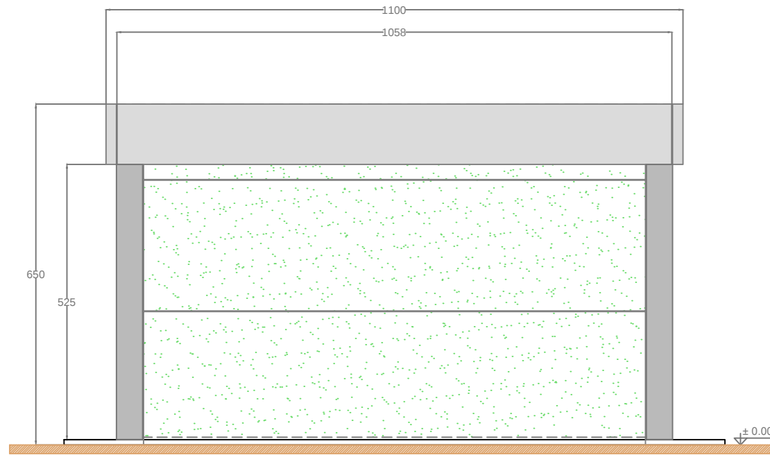
PROSPETTO D
