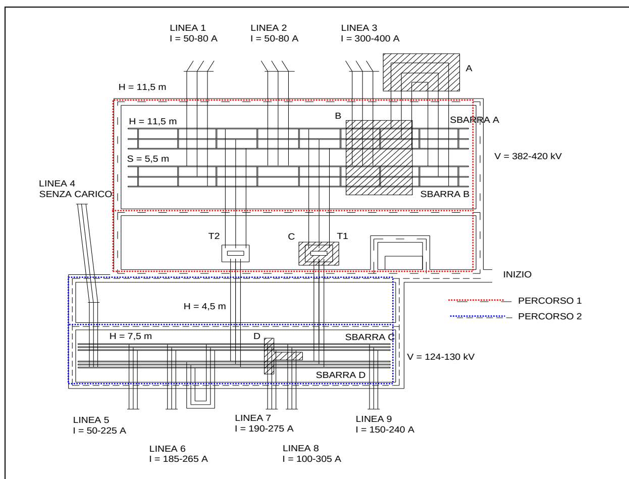
Fig. 1 Pianta di una tipica stazione 380/150 kV con indicazione delle principali distanze fase-fase (S) e fase-terra (H), nonché delle variazioni della tensione elettrica sulle sbarre e le correnti elettriche nelle varie linee aeree confluenti nella stazione durante le prove di misura di campo elettrico e magnetico.
