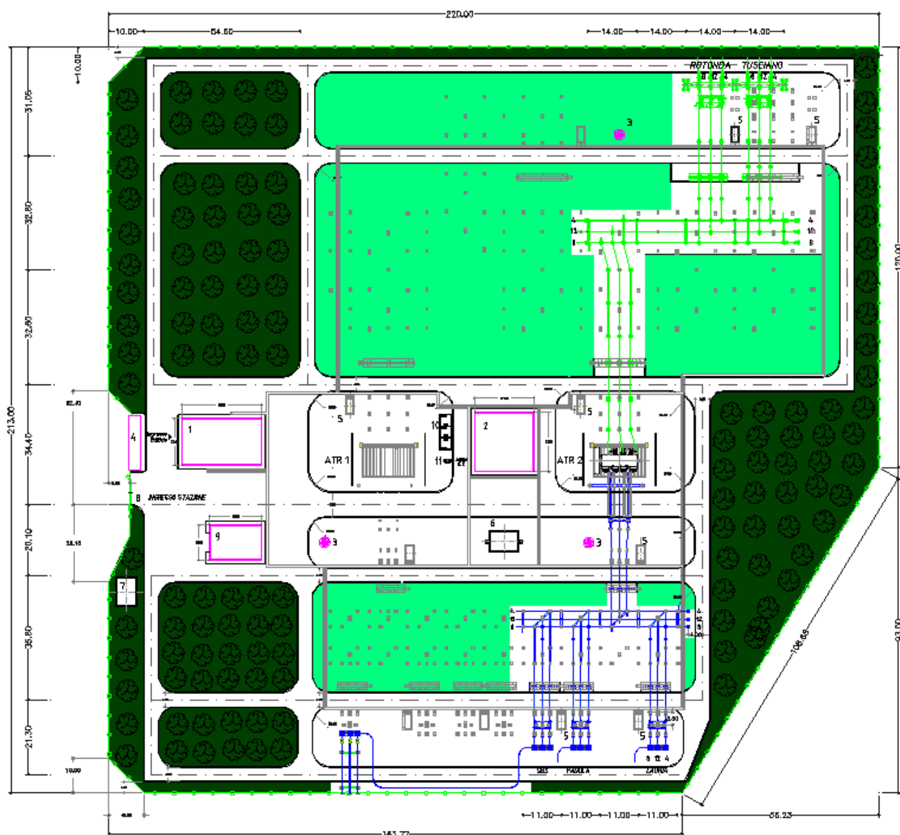
Fig.2 – Planimetria elettromeccanica generale.
