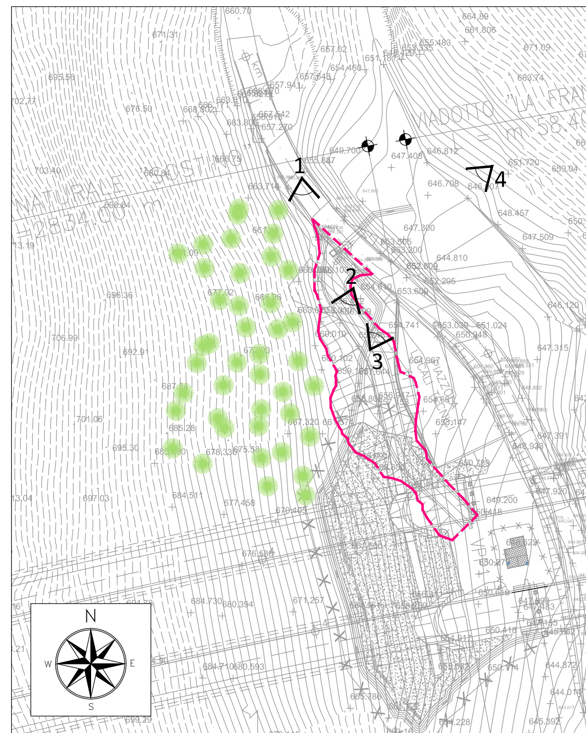
PLANIMETRIA STATO DI FATTO - SCALA 1:1000
