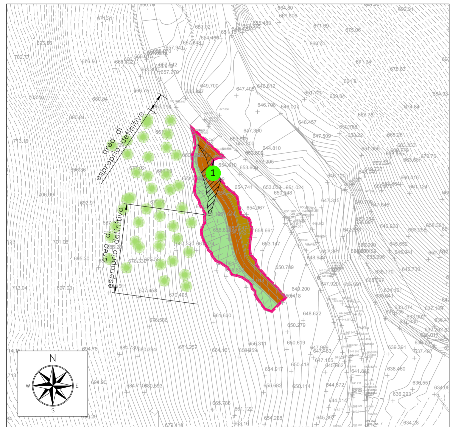
PLANIMETRIA STATO DI FATTO - SCALA 1:1000
