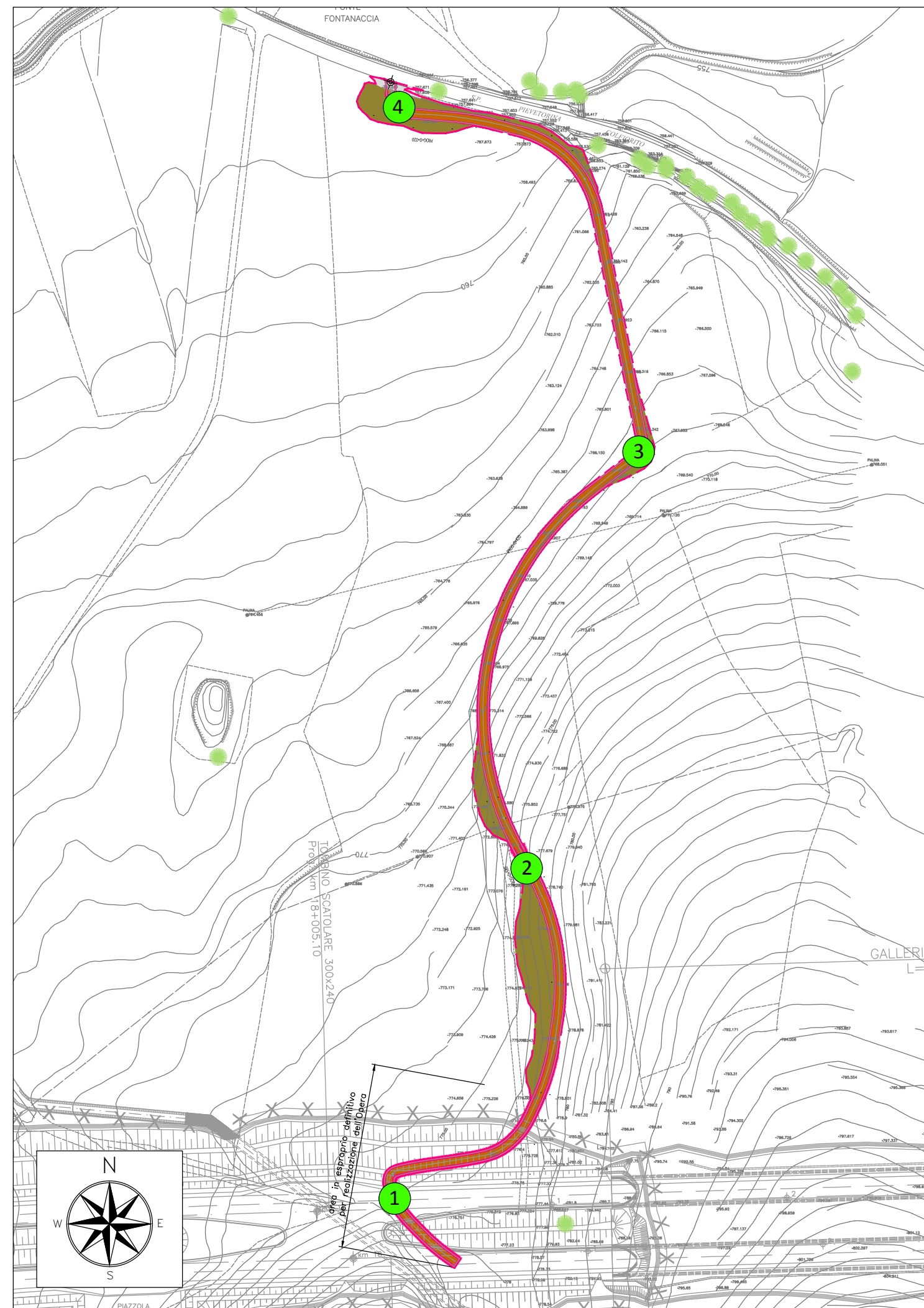
PLANIMETRIA STATO DI FATTO - SCALA 1:1000
