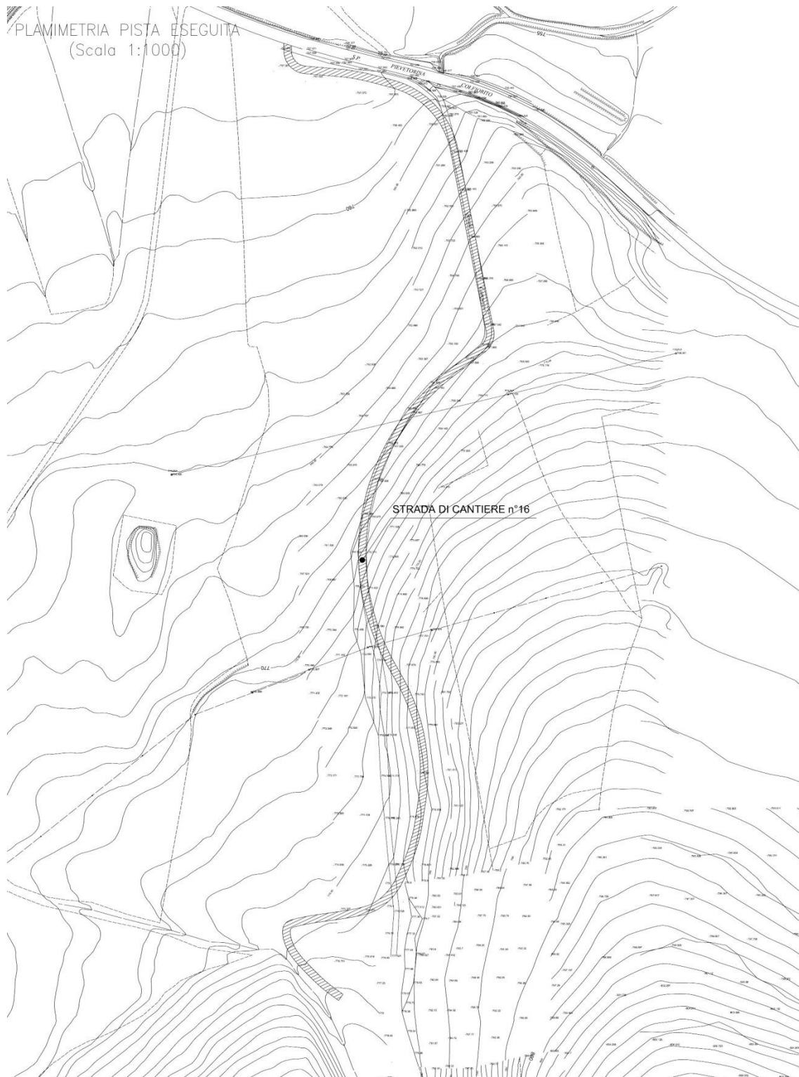
Figura 1 – Progetto pista di cantiere
