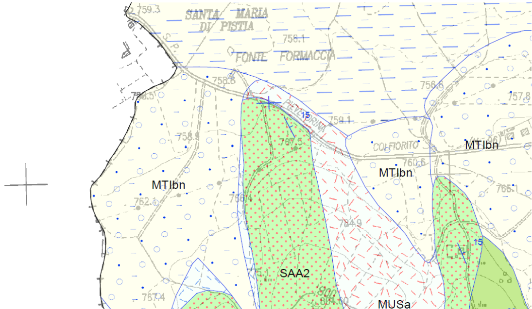
Figura 4 – Stralcio della Carta geologica regionale dell'area - stralcio Sezione 312150
