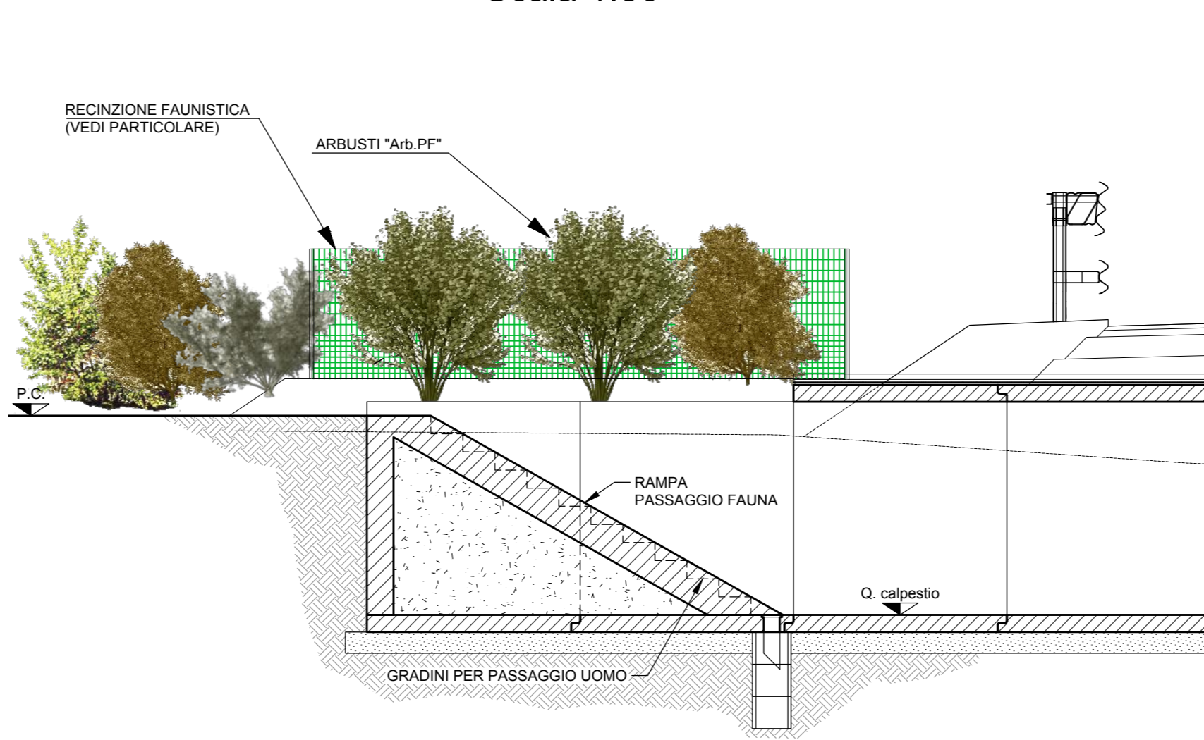
PASSAGGIO FAUNA SEZIONE LONGITUDINALE Scala 1:50
