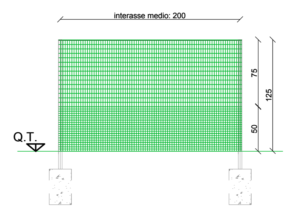
PARTICOLARE RECINZIONE FAUNISTICA Scala 1:25
