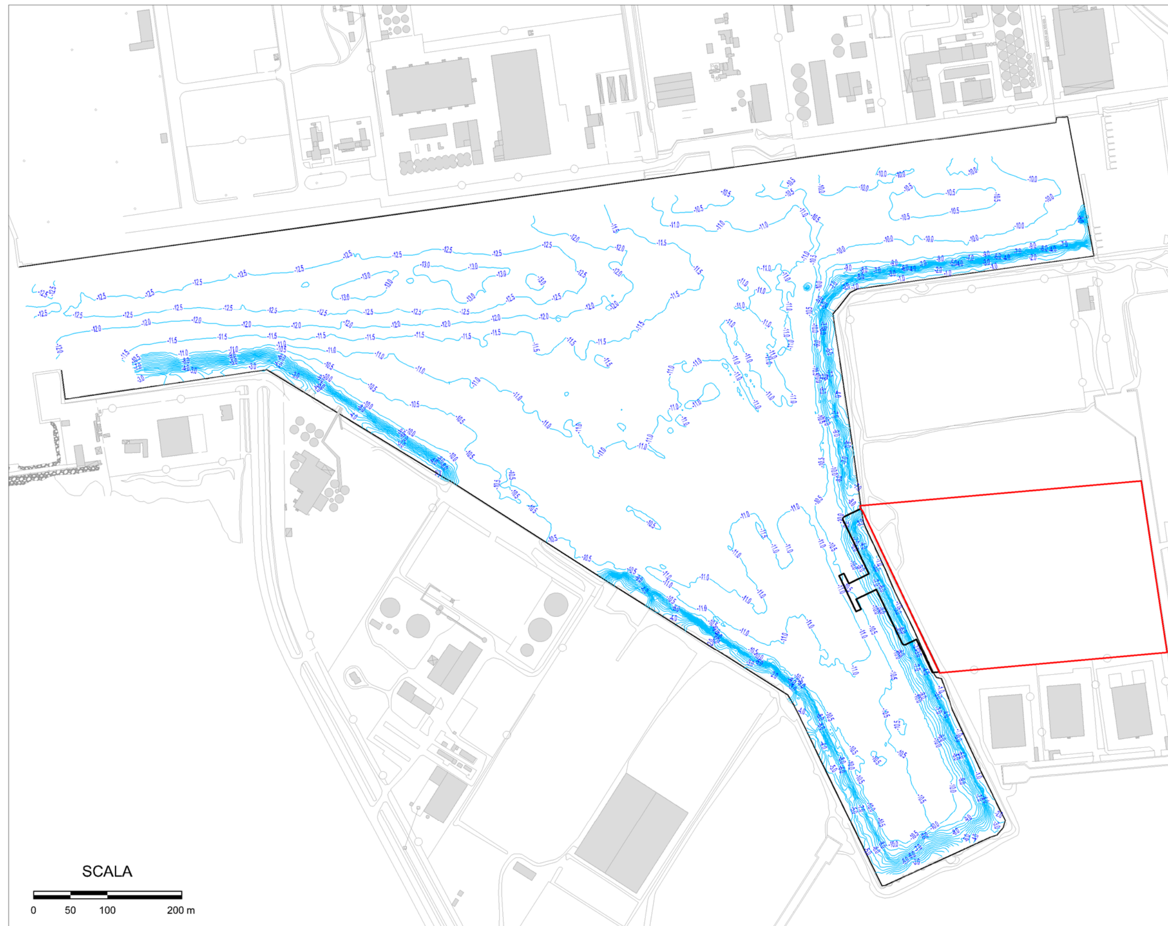
BATIMETRIA DEL BACINO PORTUALE (SURVEY BATIMETRICO MAGGIO 2015)
