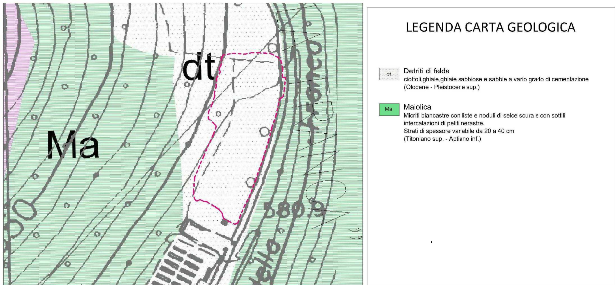
Figura 5 – Stralcio della Carta geologica dell'area e relativa legenda
